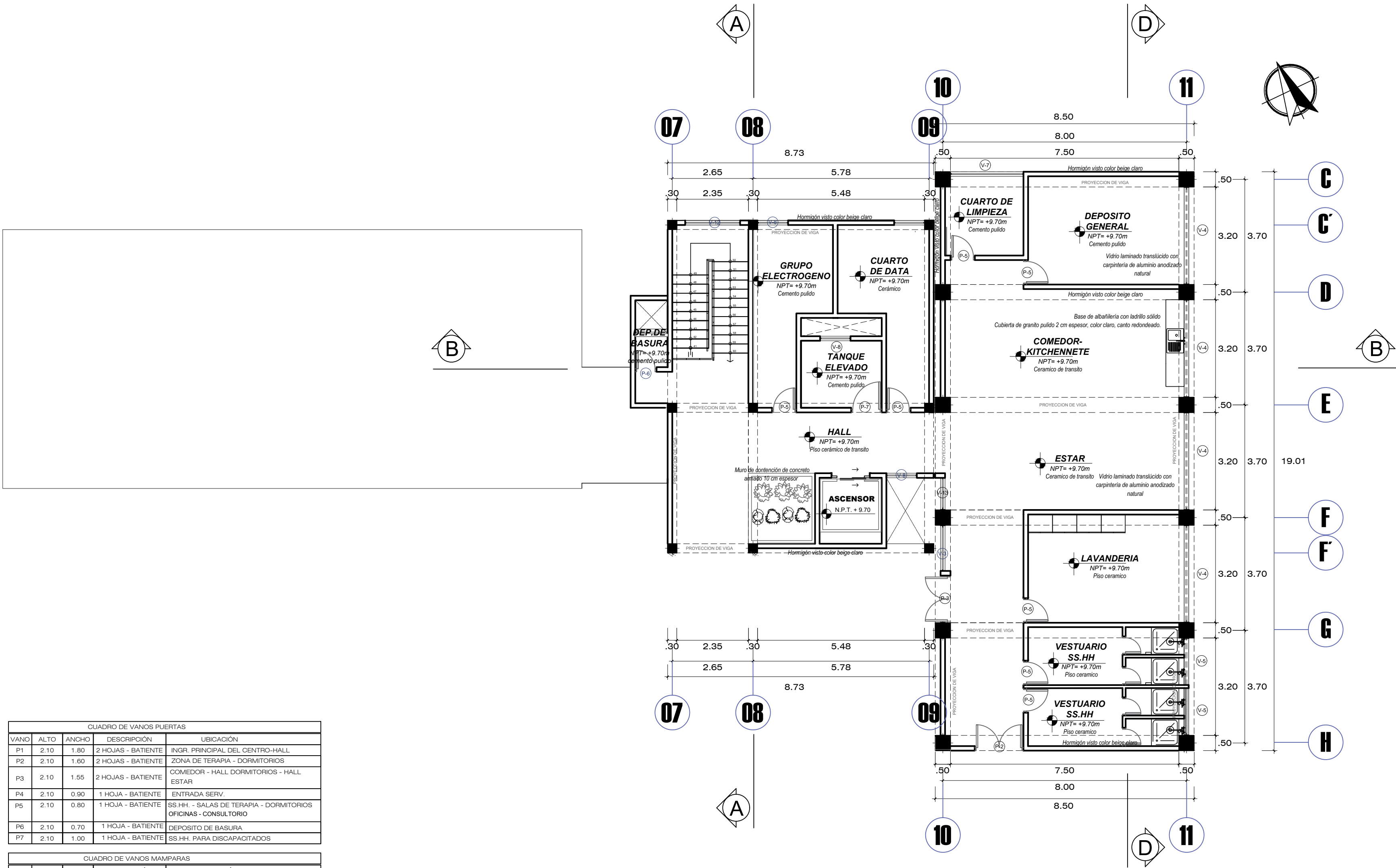
PLANIMETRIA DE DISTRIBUCION - 4TO NIVEL ESCALA = 1/100
