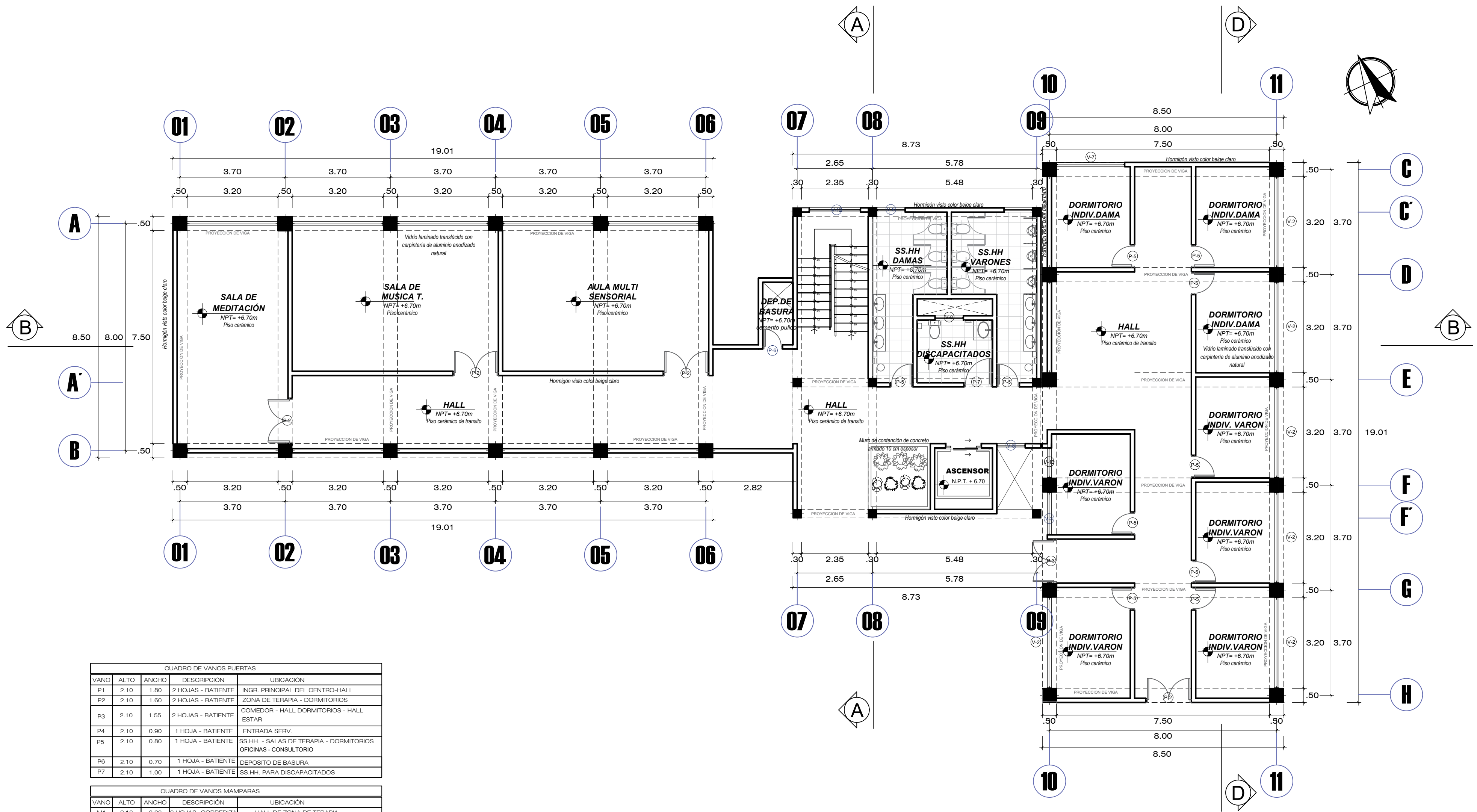
PLANIMETRIA DE DISTRIBUCION - 3ER NIVEL ESCALA = 1/100
