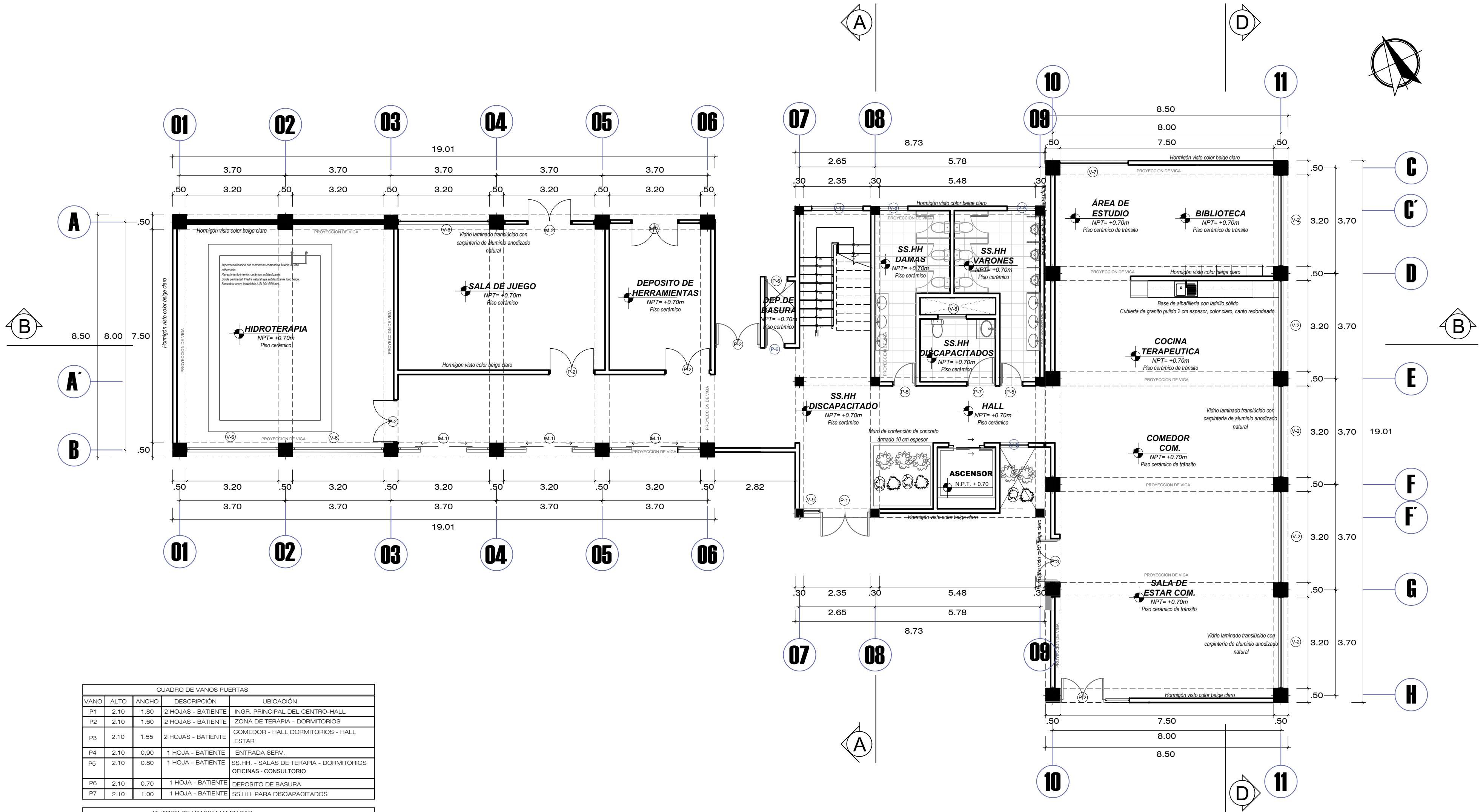
PLANIMETRIA DE DISTRIBUCION - 1ER NIVEL ESCALA = 1/100
