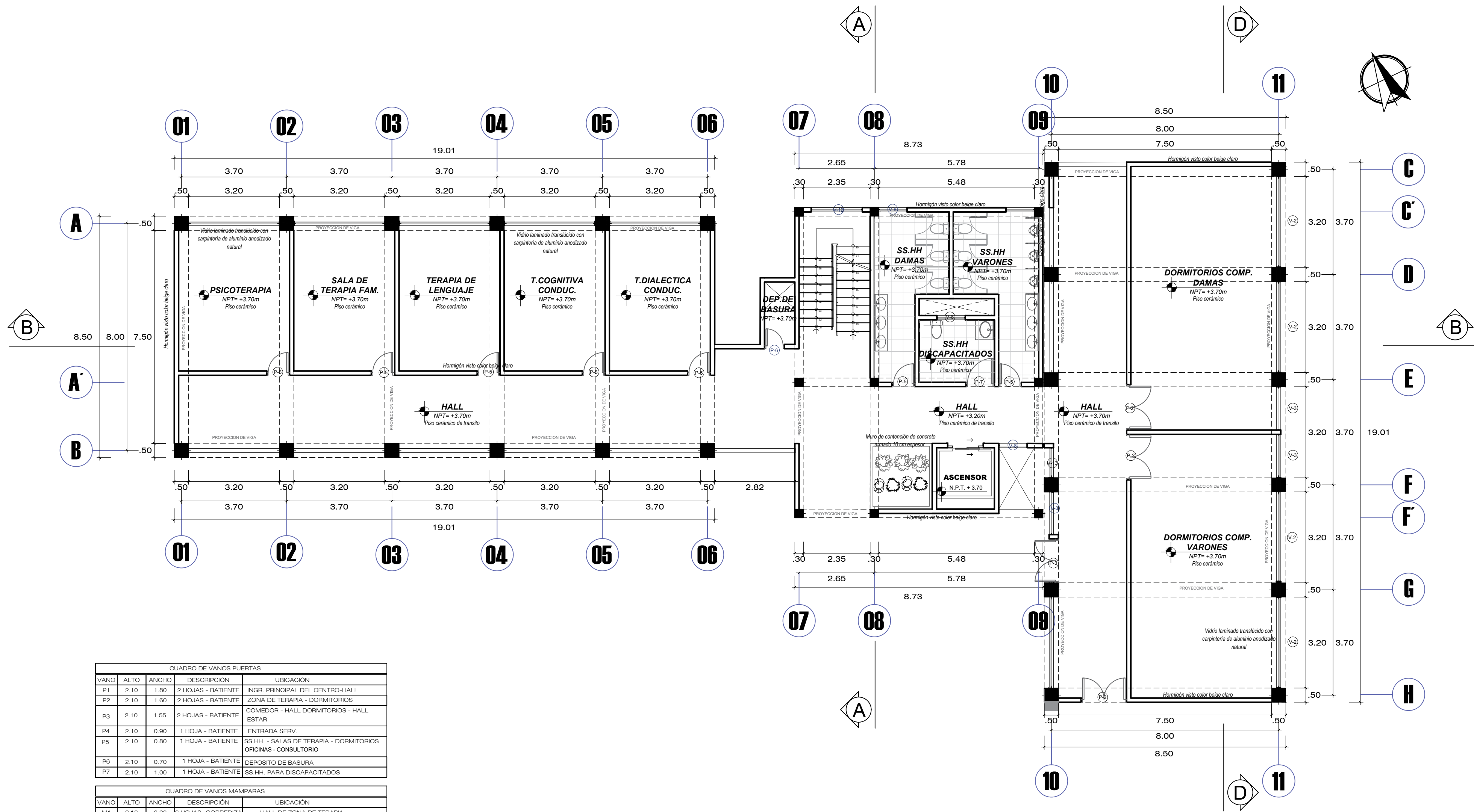
PLANIMETRIA DE DISTRIBUCION - 2DO NIVEL ESCALA = 1/100
