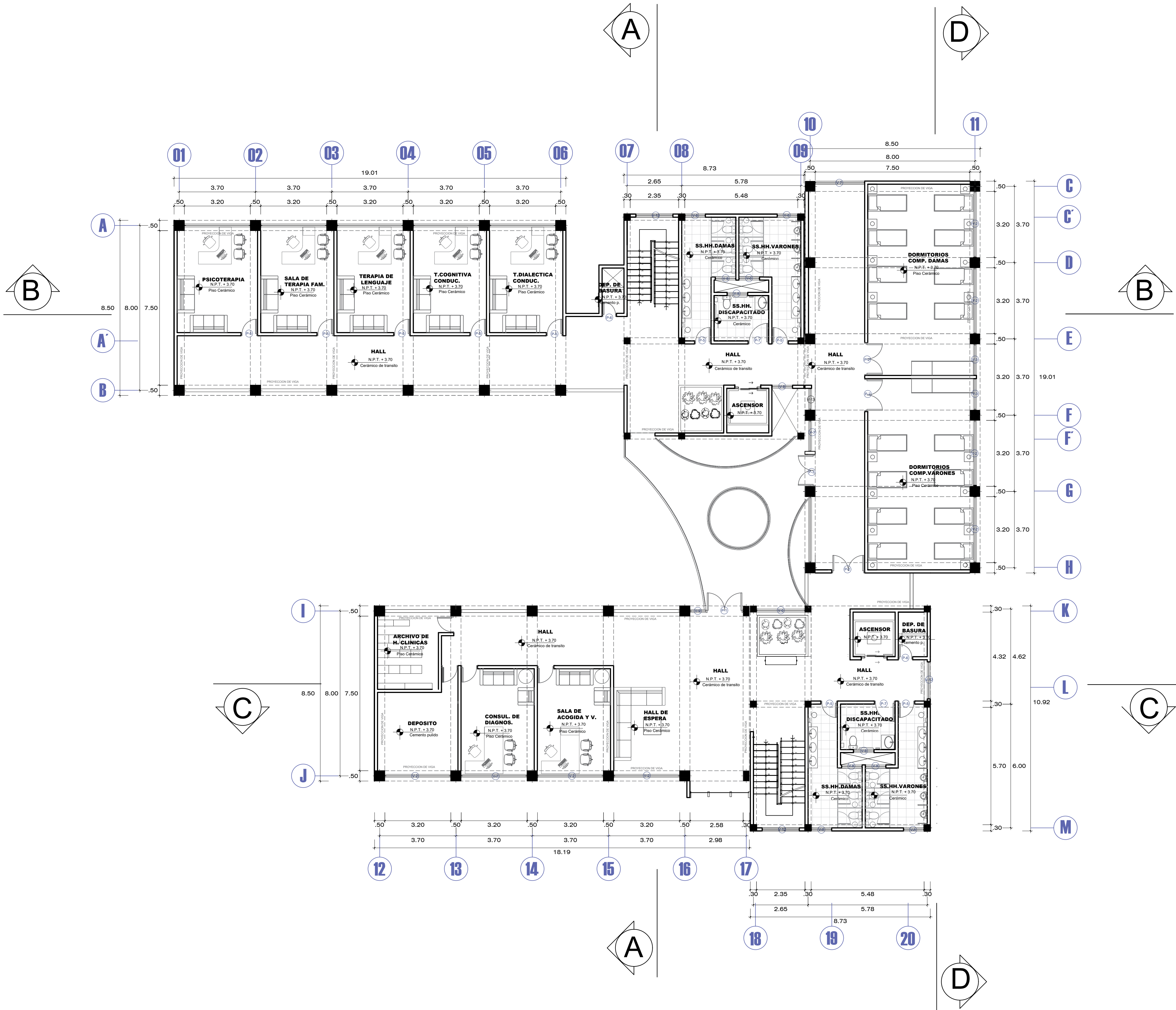
PLANO DE DISTRIBUCION SEGUNDO PISO esc. 1/100
