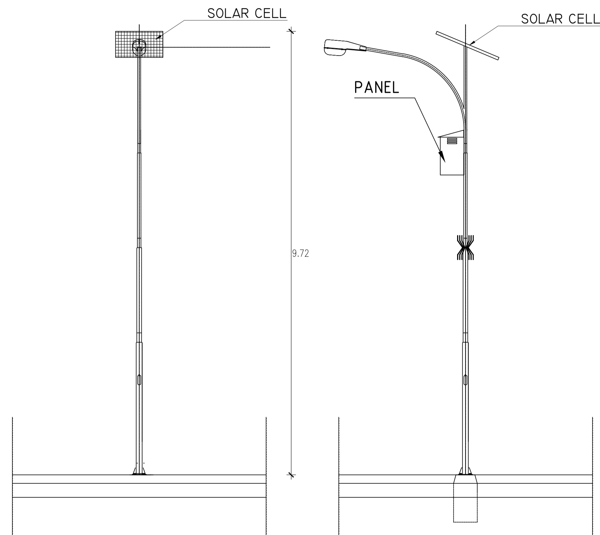
DETALLE DE POSTE CON PANEL SOLAR NTS
