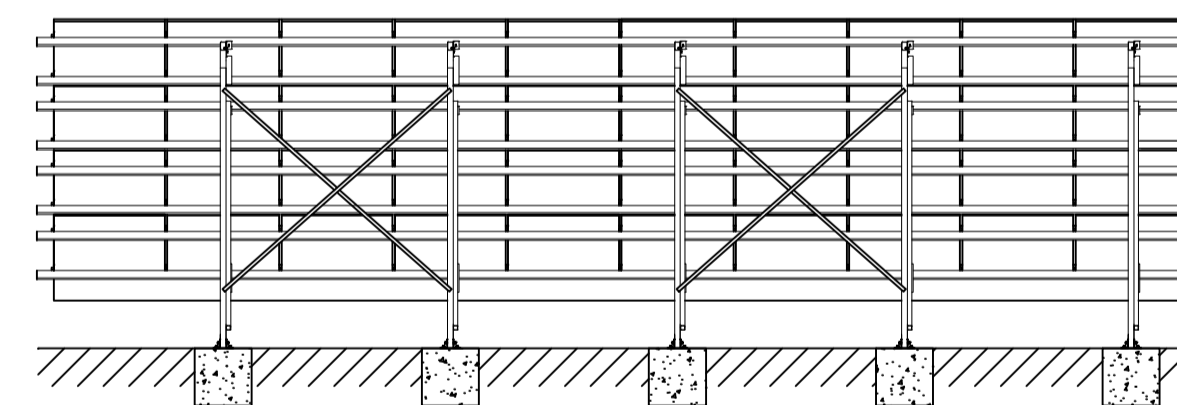
VISTA TRASERA DE PANEL SOLAR NTS
