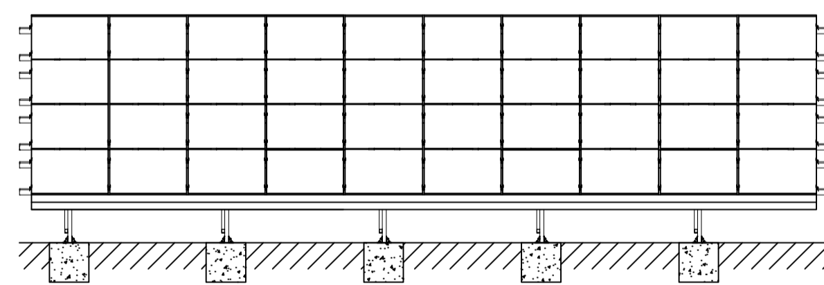
VISTA FRONTAL DE PANEL SOLAR NTS
