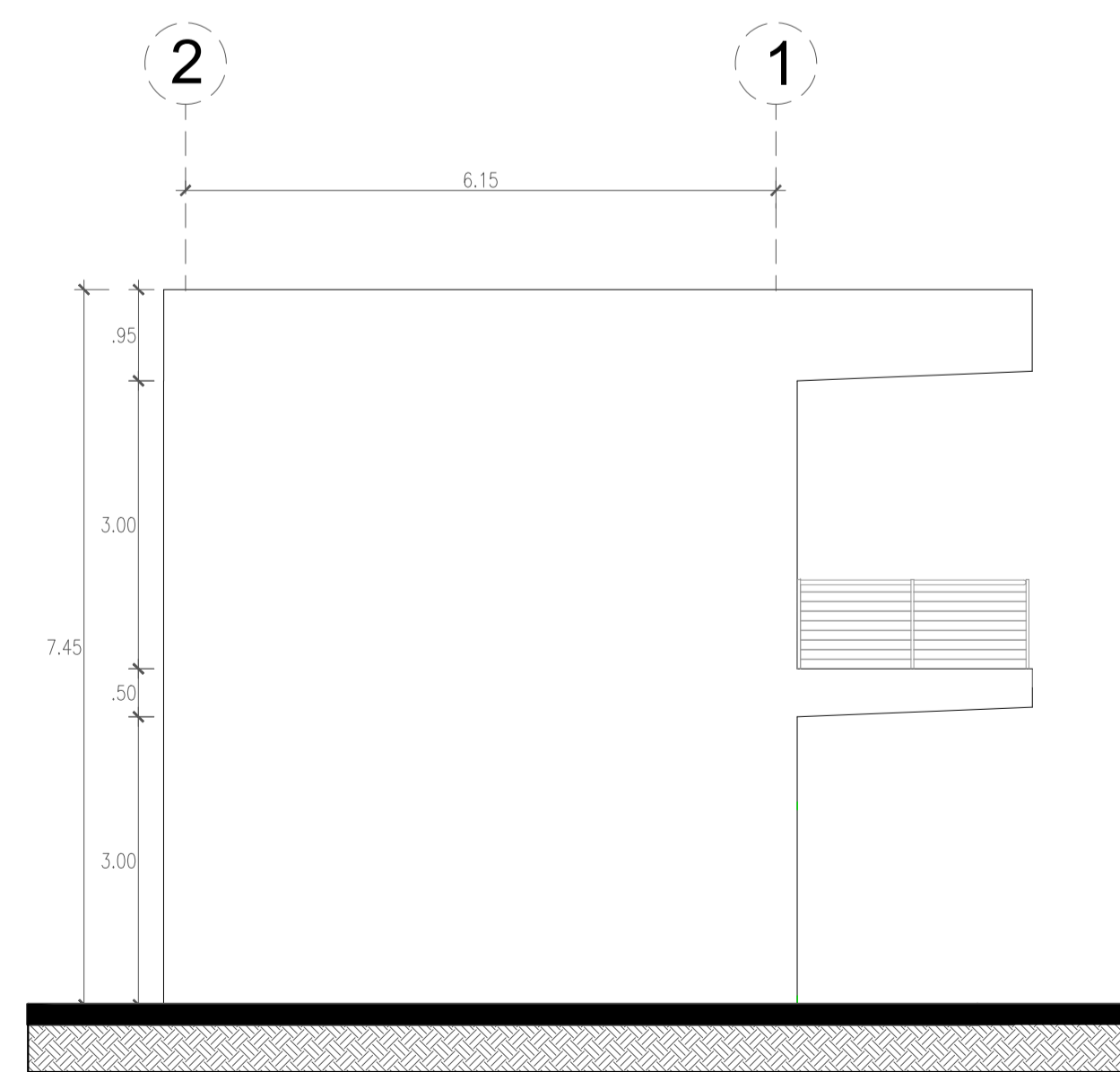
BLOQUE D - ELEVACION LATERAL IZQUIERDA Elev. 1/80
