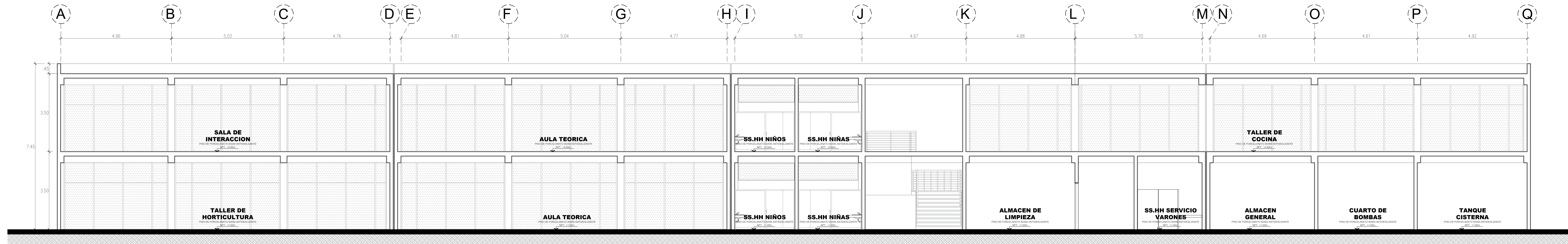
BLOQUE D - CORTE A-A Escala: 1/50
