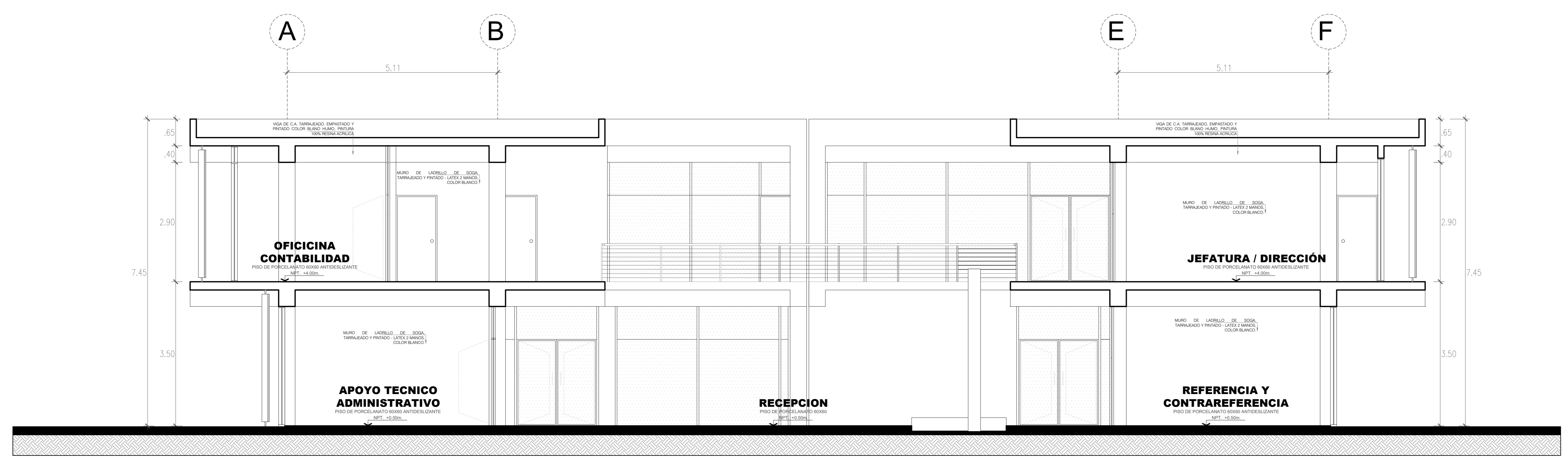
BLOQUE A - CORTE B-B Escala: 1/80
