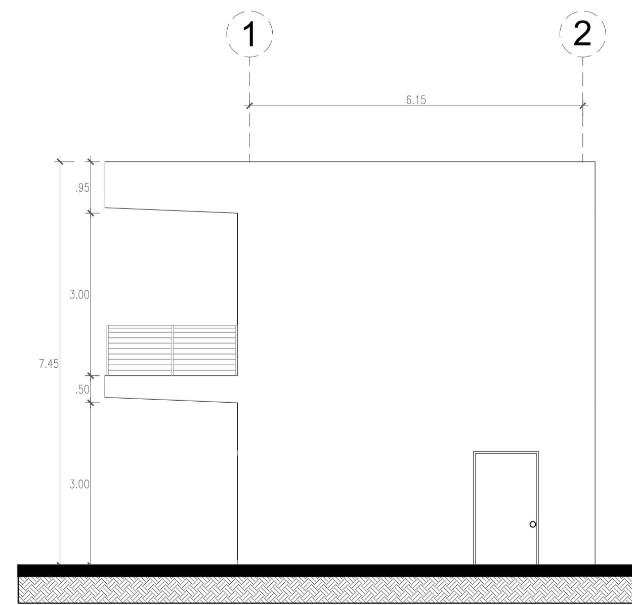
BLOQUE D - ELEVACION LATERAL DERECHA Elev. 1/80
