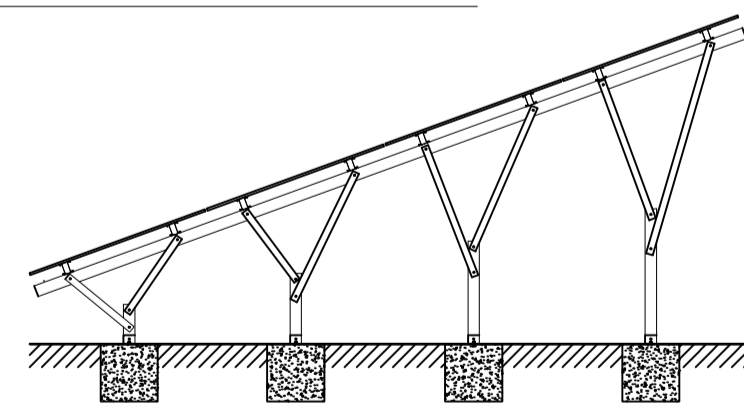
VISTA LATERAL DE PANEL SOLAR NTS
