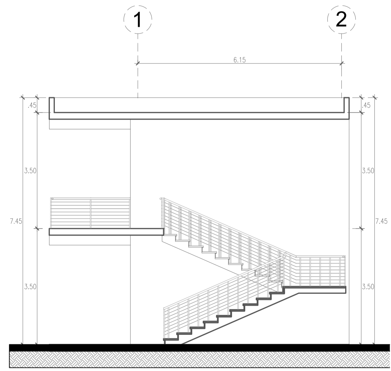
BLOQUE D - CORTE B-B Escala: 1/50
