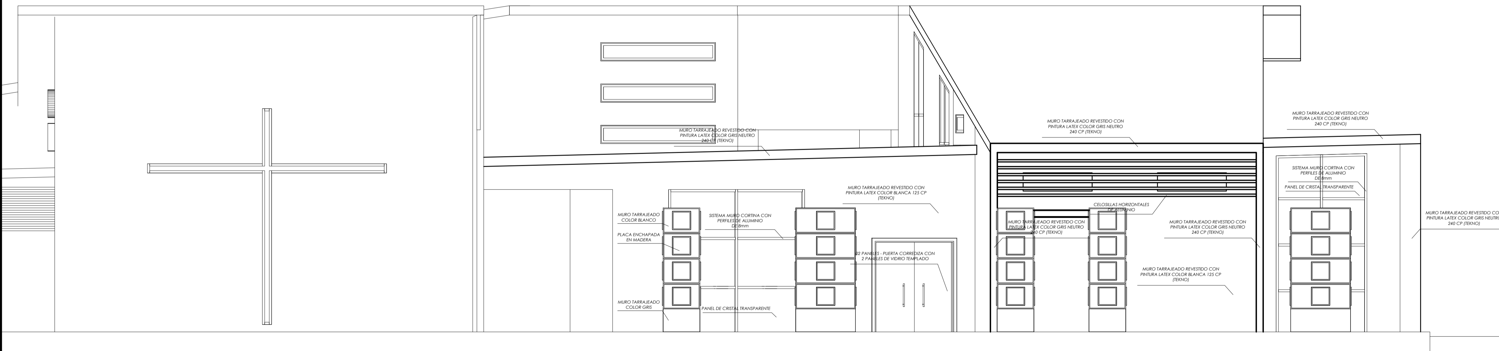
ELEVACION LATERAL Esc. 1/50
