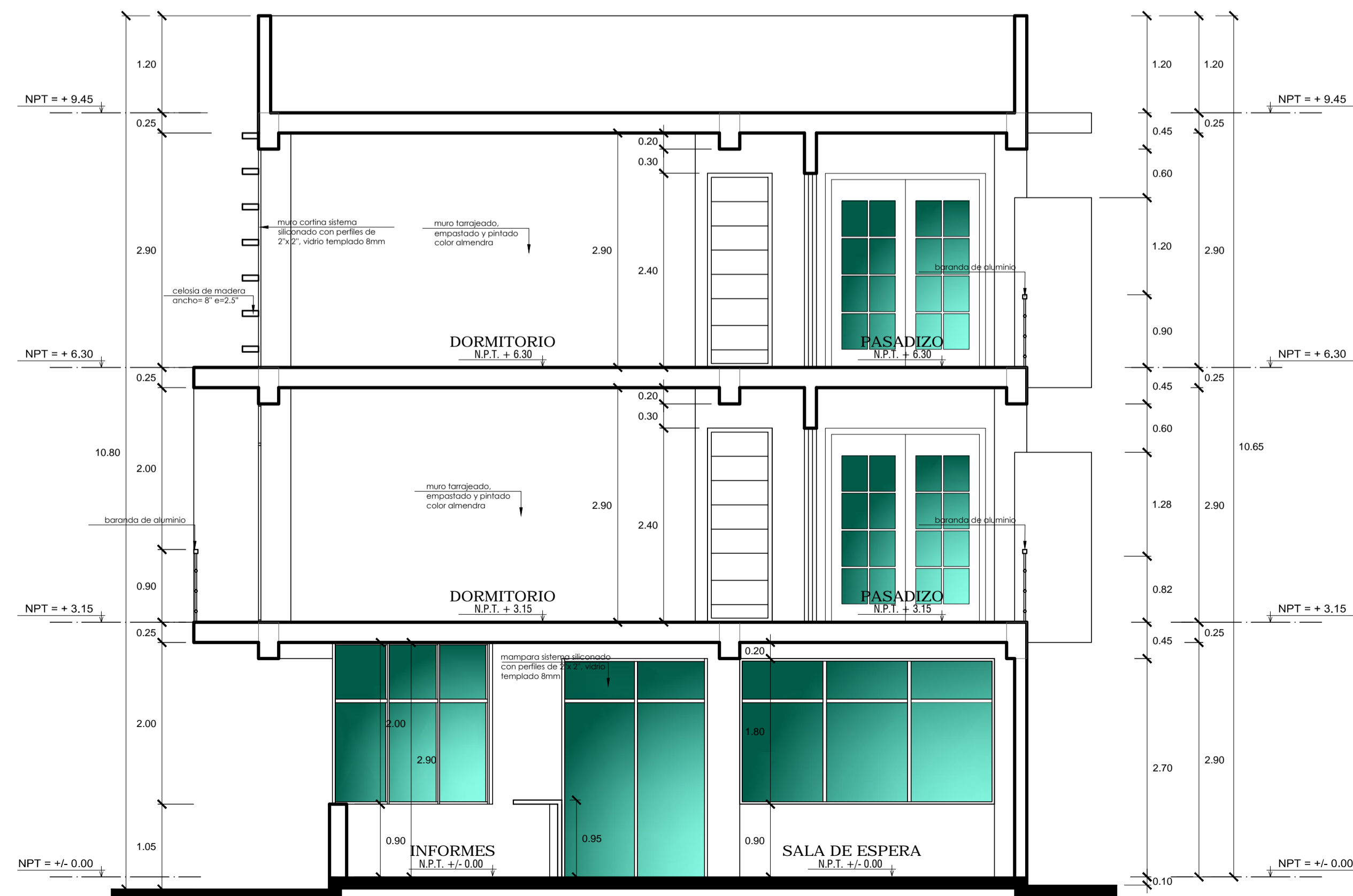
CORTE D - D esc:1/50
