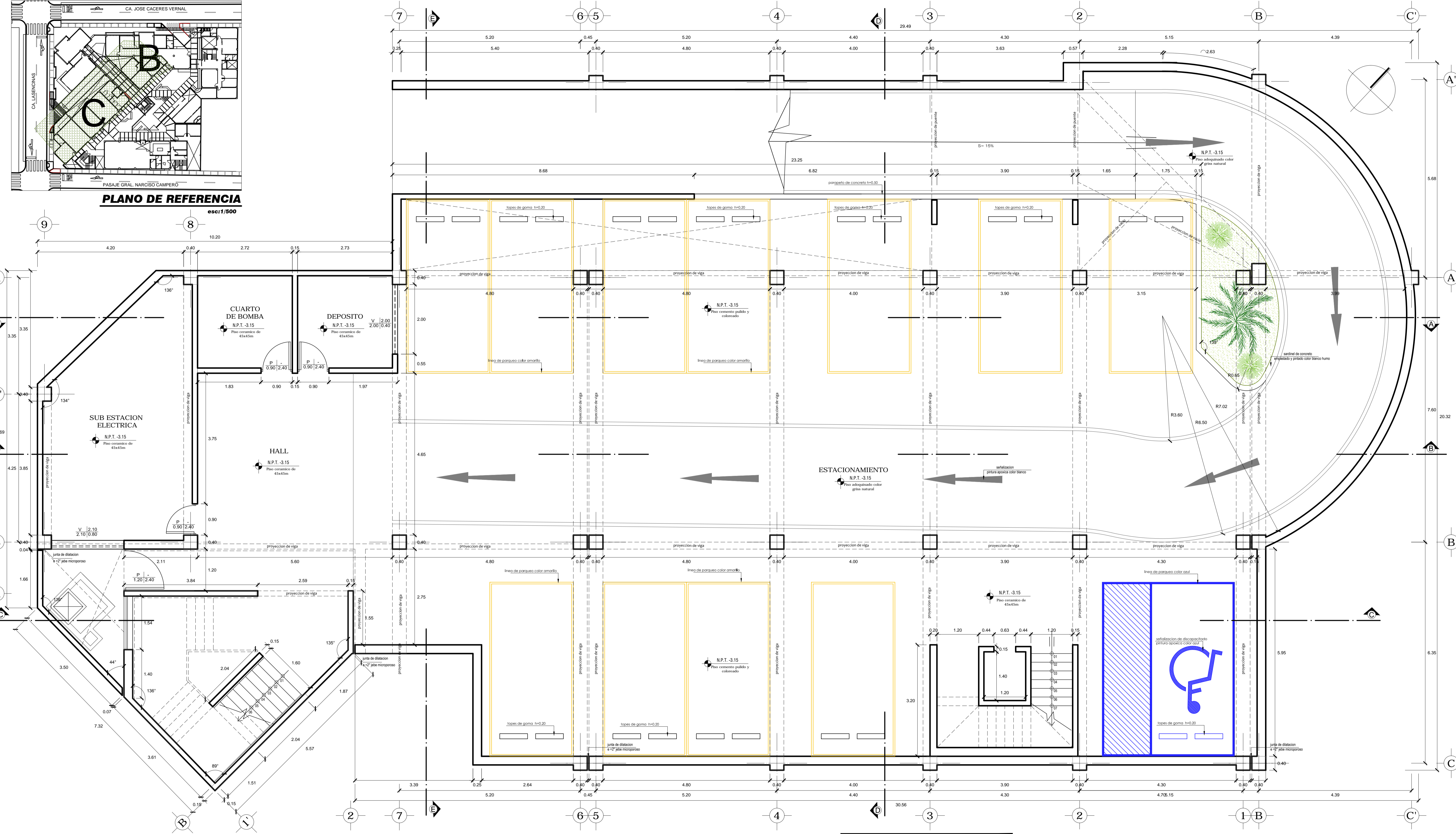
PLANTA DE SOTANO esc:1/50
