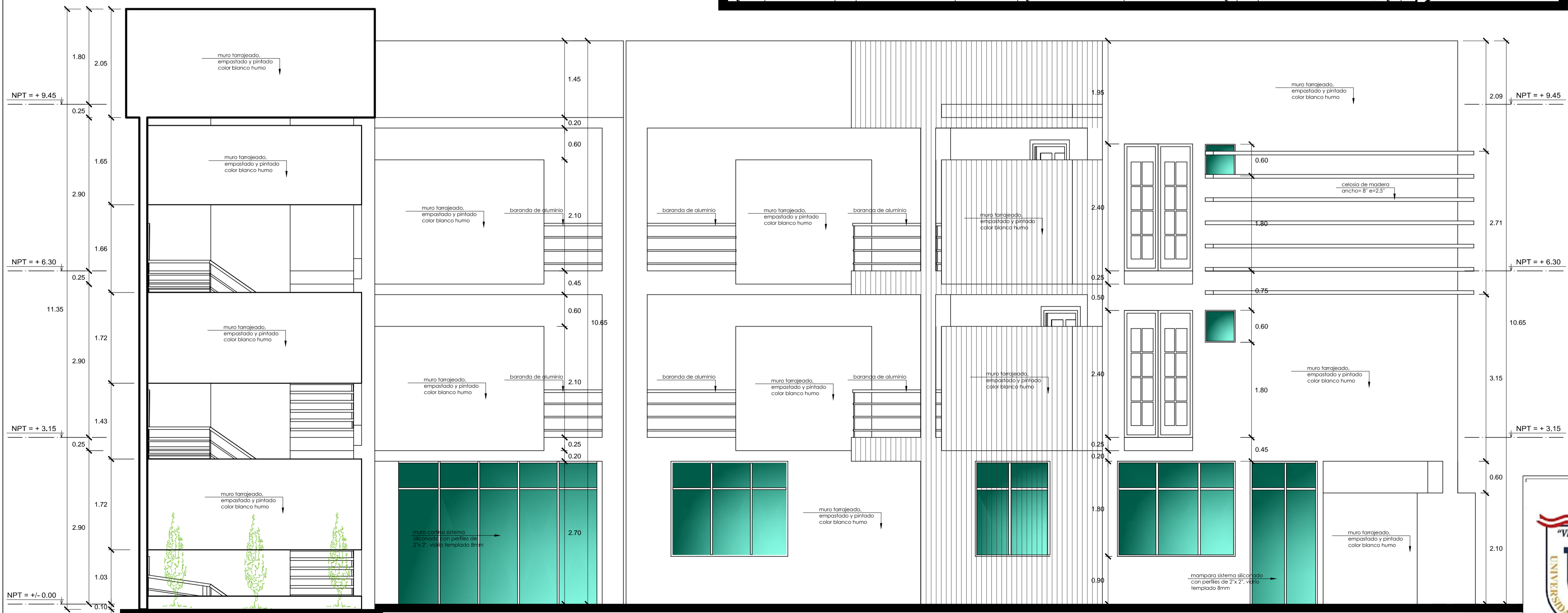
ELEVACION LATERAL E-1 esc:1/50
