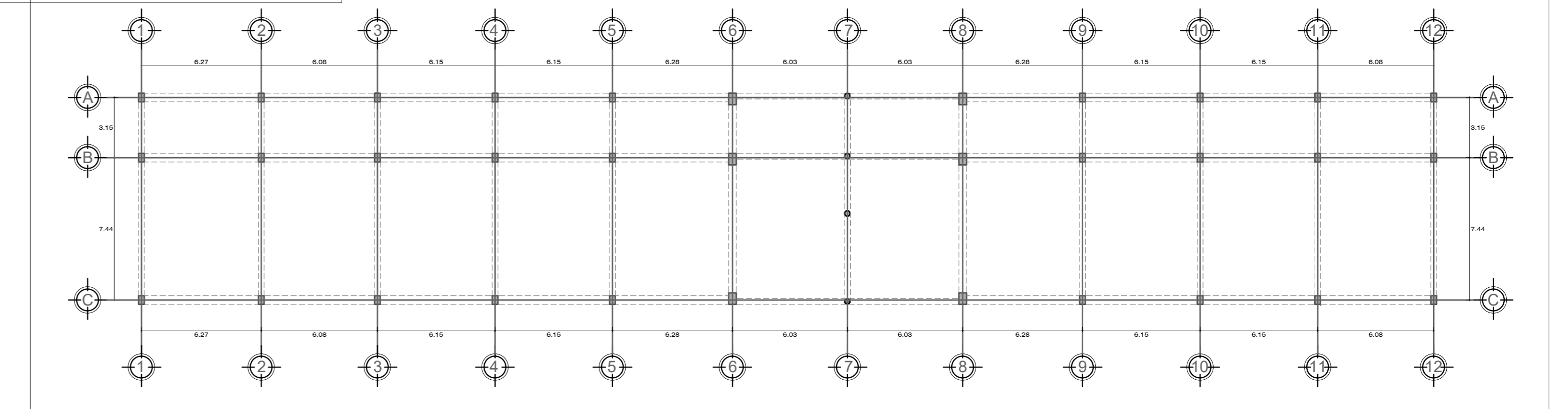
PLANO ESTRUCTURAS - SECTOR 2 PORTICOS DUCTILES ESC:1/200
