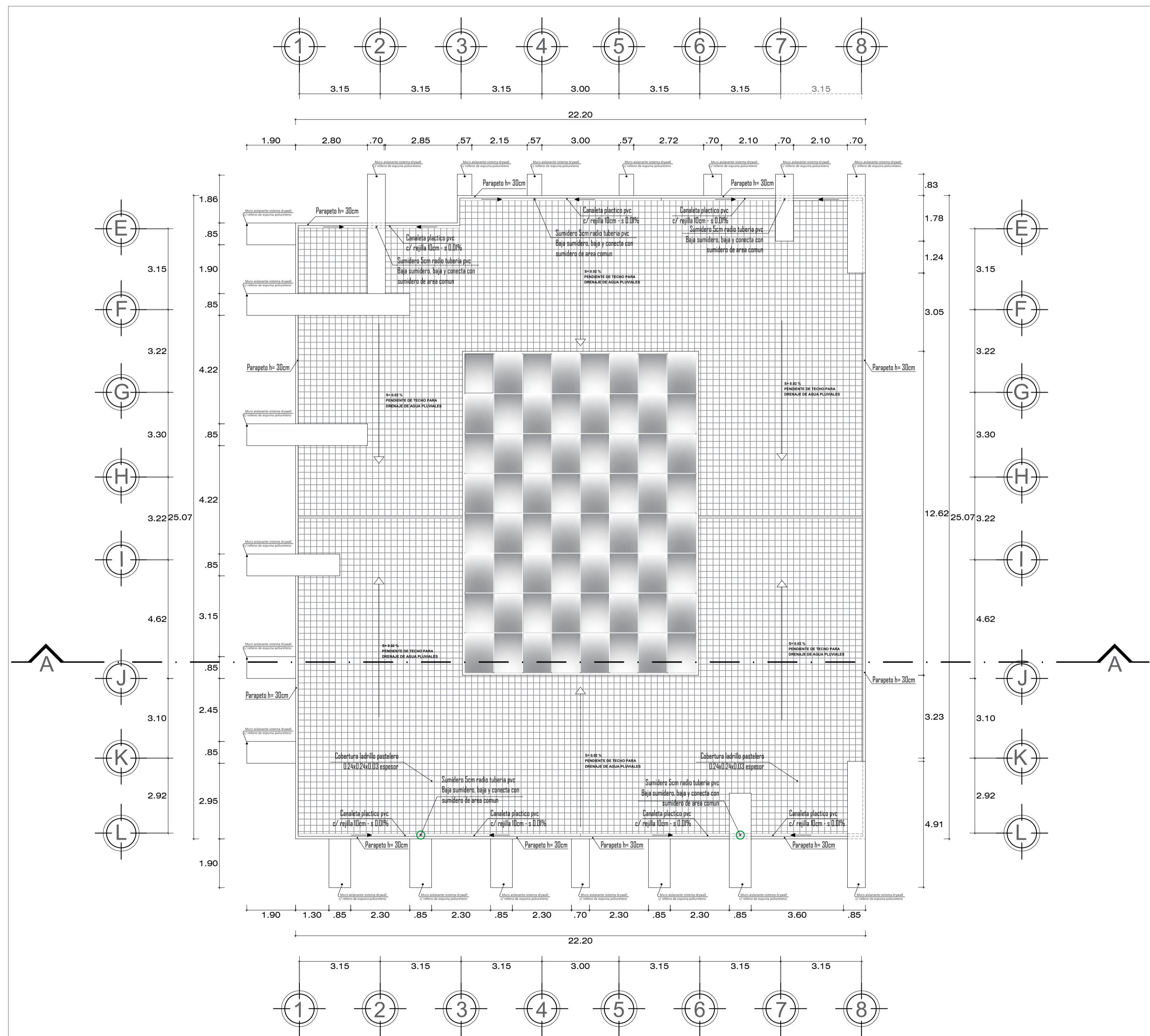
SECTOR - 1: PLANO DE TECHOS PROYECTO escala 1:75
