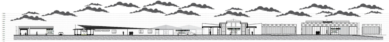
CORTE C-C' PLANIMETRIA GENERAL ESC.1/250
