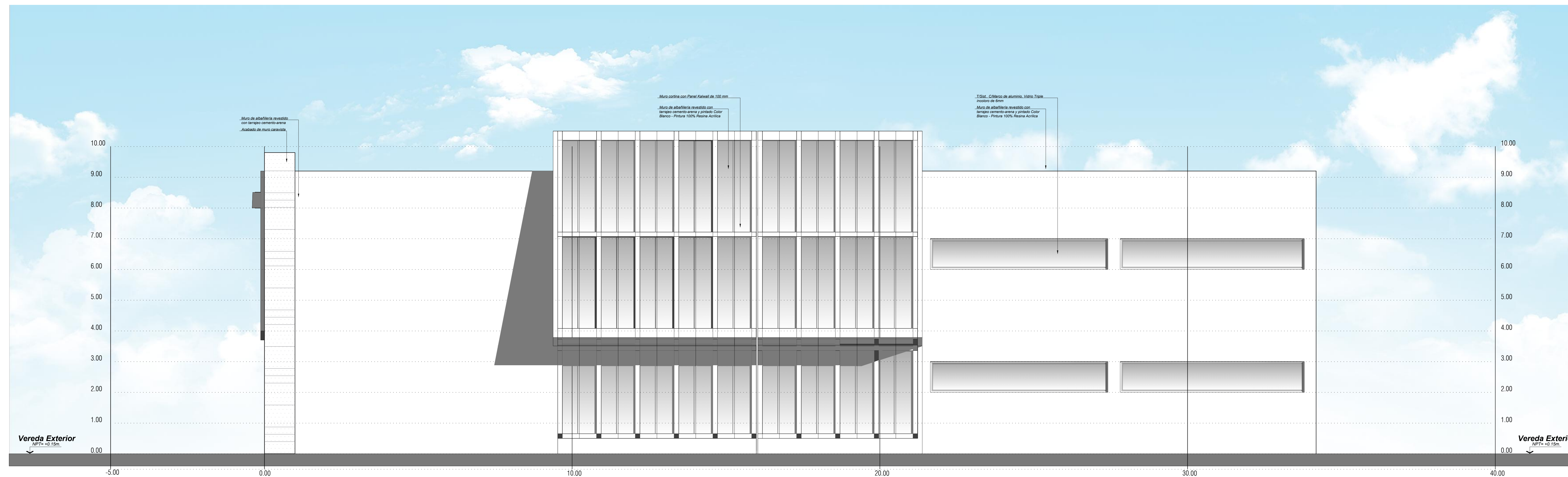
ARQUITECTURA ELEVACIÓN E - 2 esc. 1/50 BLOQUE 01- 02
