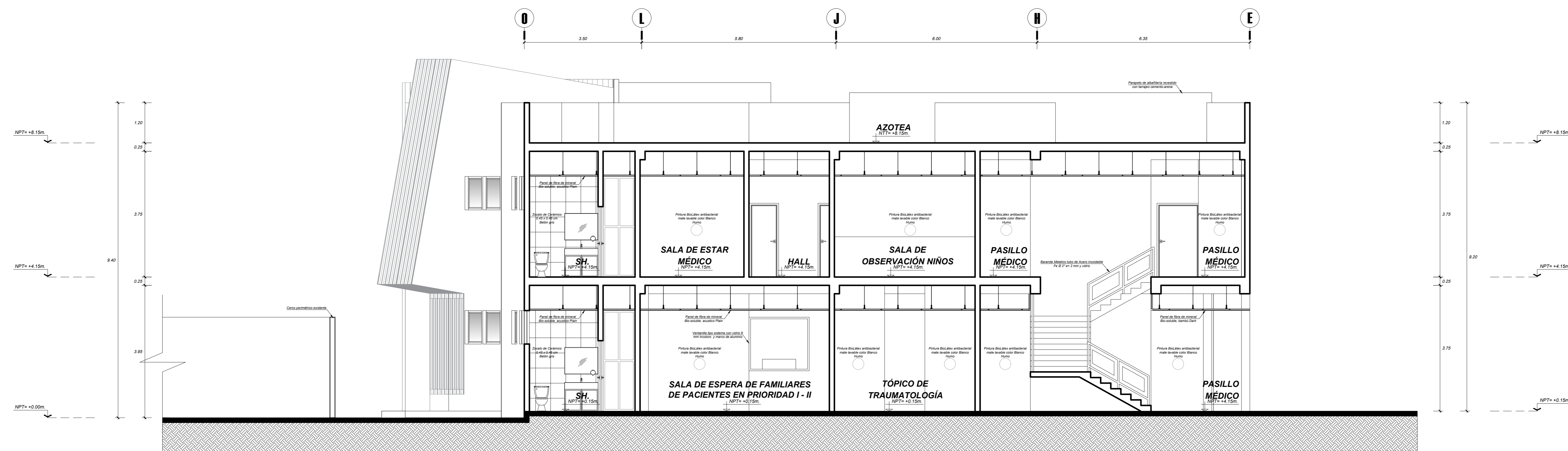
CORTE B - B esc. 1/50 BLOQUE 03
