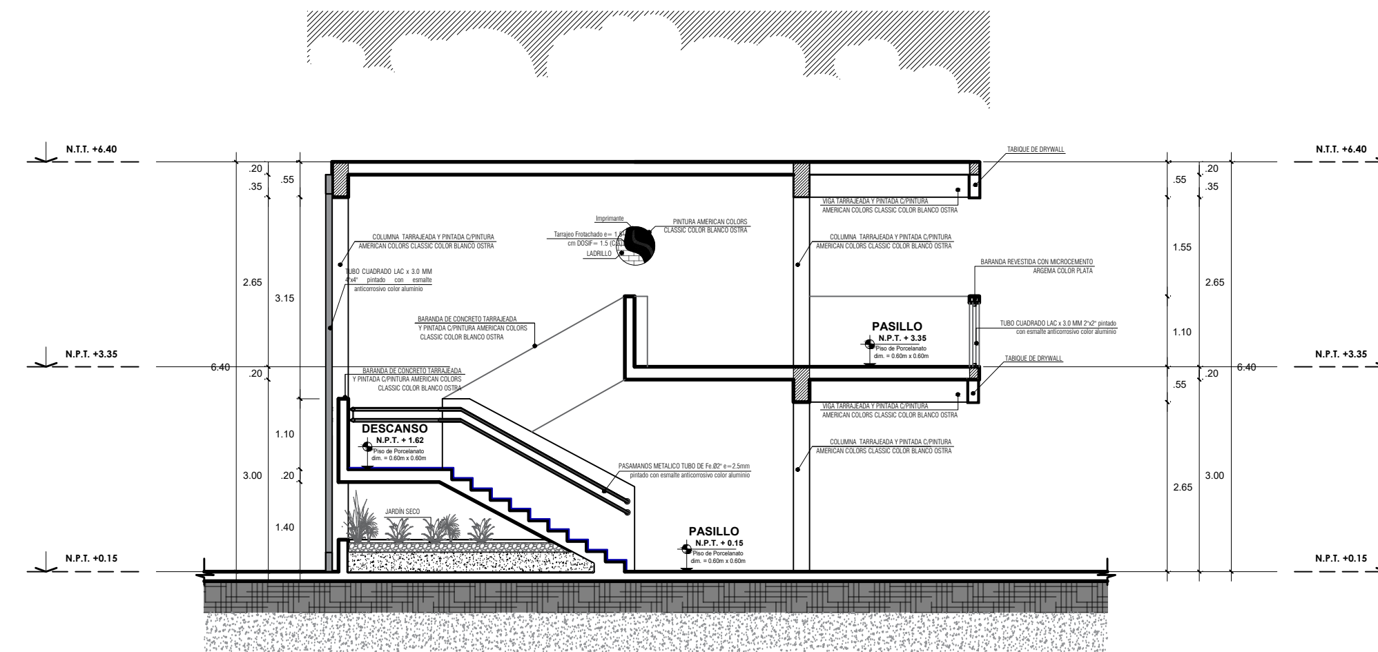
CORTE B-B' - BLOQUE 08 ESCALA 1/75
