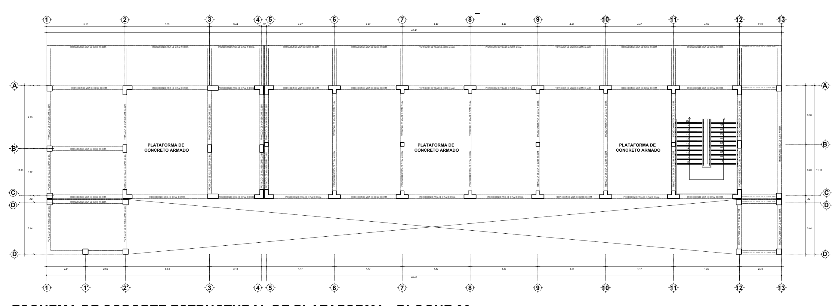
ESQUEMA DE SOPORTE ESTRUCTURAL DE PLATAFORMA - BLOQUE 06 ESCALA 1/150
