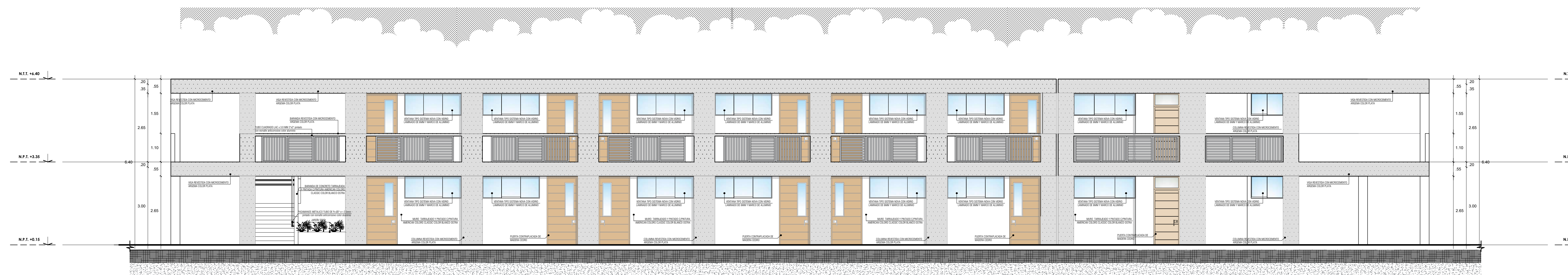
ELEVACIÓN 01 - BLOQUE 06 ESCALA 1/75
