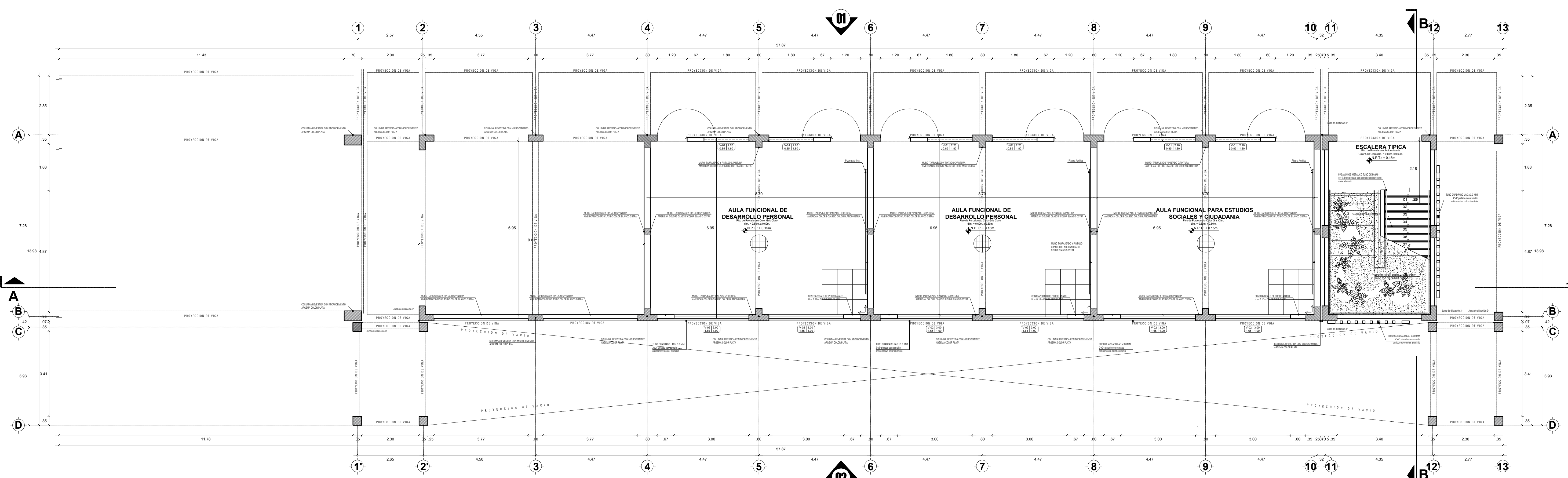
PRIMER NIVEL - BLOQUE 08 ESCALA 1/75
