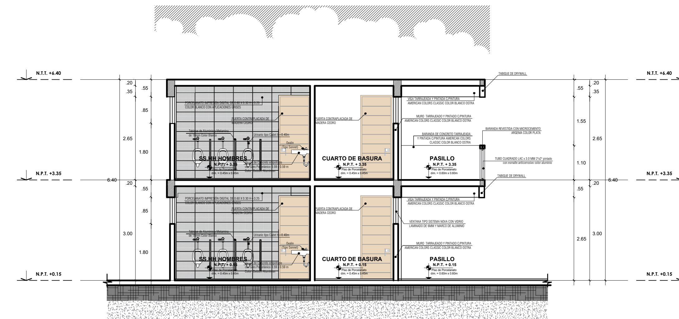
CORTE B-B' - BLOQUE 06 ESCALA 1/75
