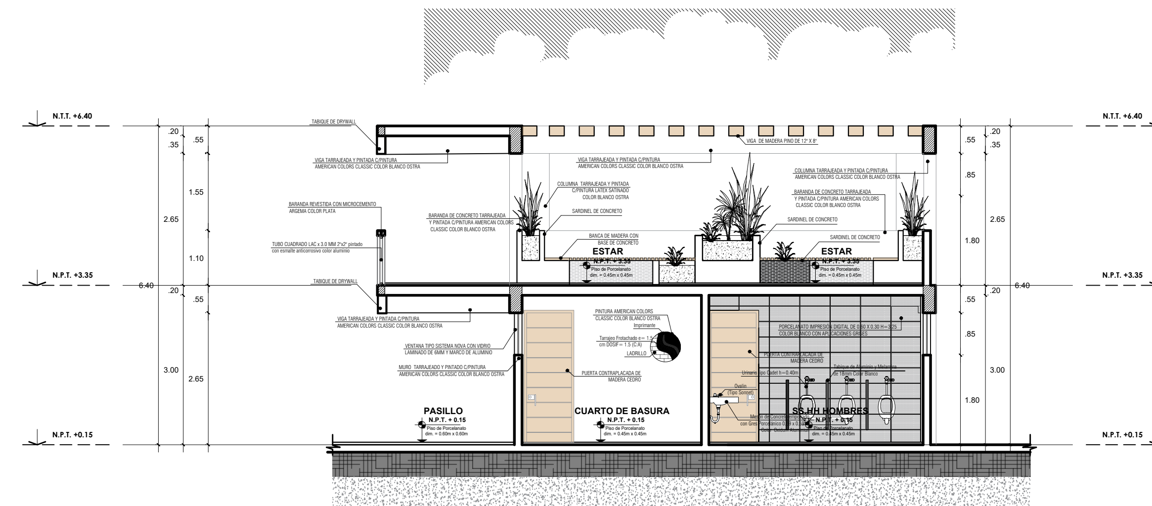
CORTE B-B' - BLOQUE 07
