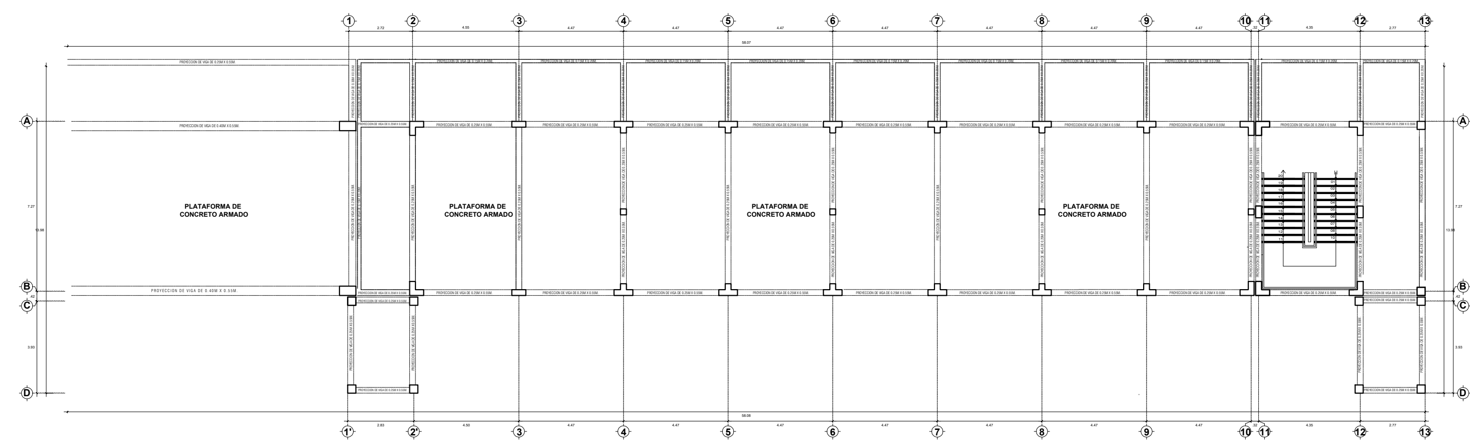
ESQUEMA DE SOPORTE ESTRUCTURAL DE PLATAFORMA - BLOQUE 08 ESCALA 1/50
