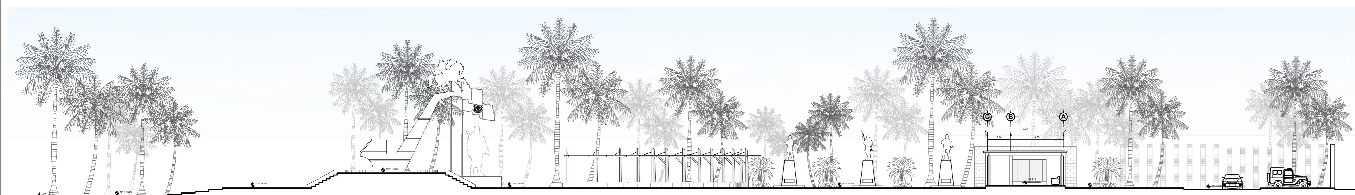
CORTE B - B' ESCALA 1/100
