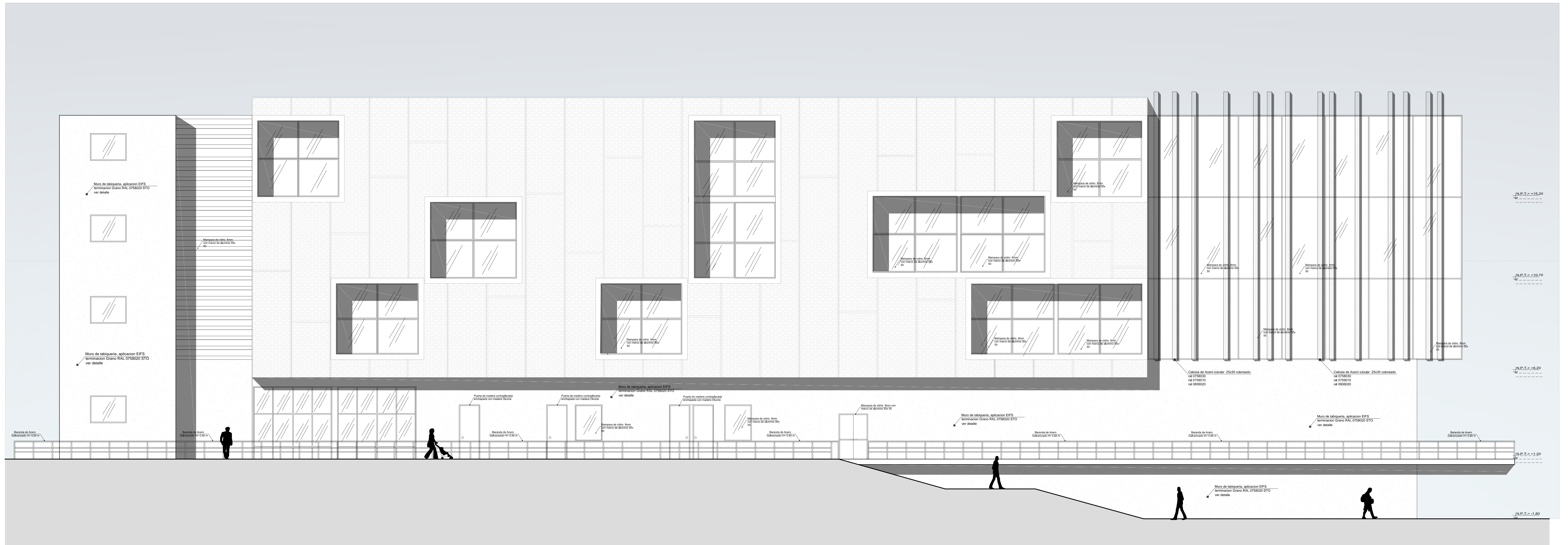
Plano : ELEVACION FRONTAL CENTRO COMERCIAL ZOFRA TACNA
