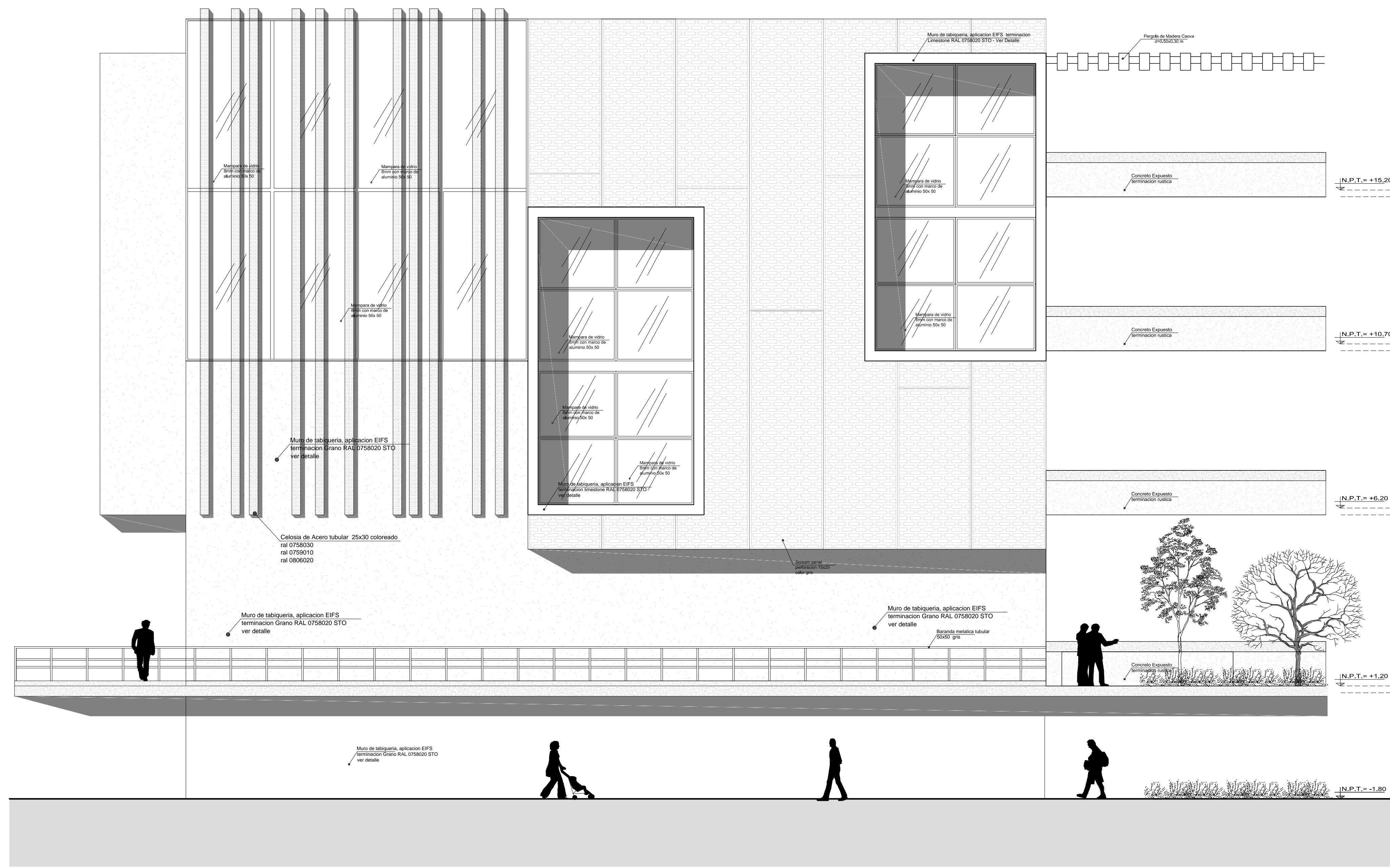
Plano : ELEVACION LATERAL DERECHO CENTRO COMERCIAL ZOFRA TACNA
