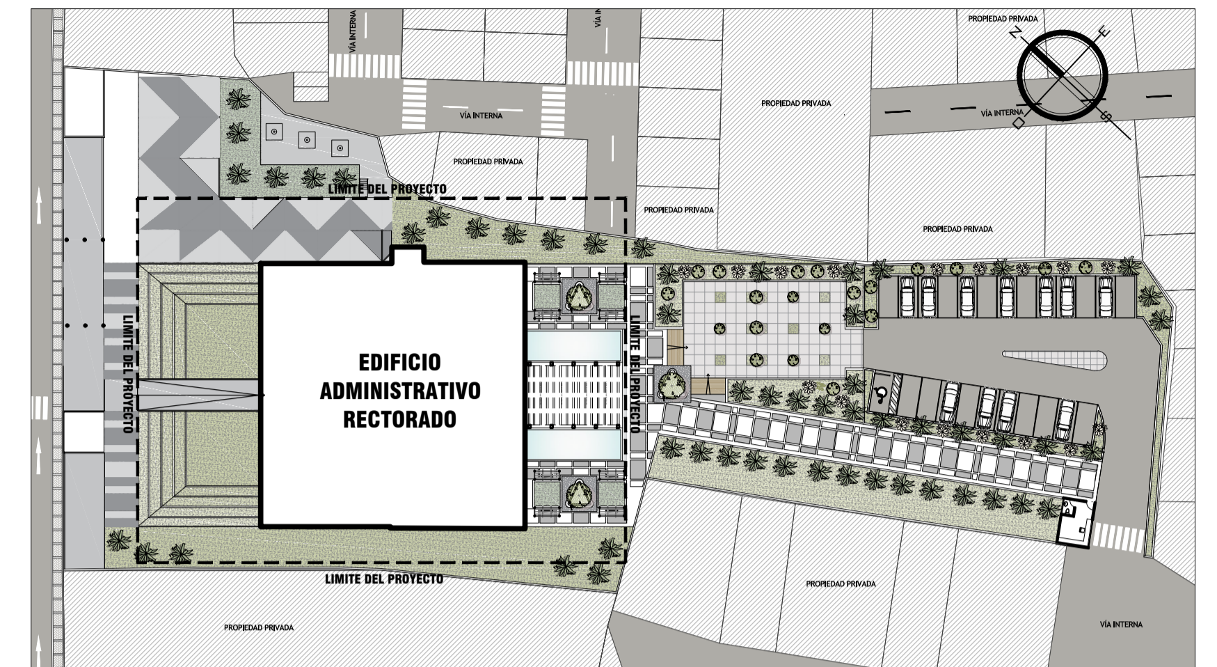
PLANO CLAVE
