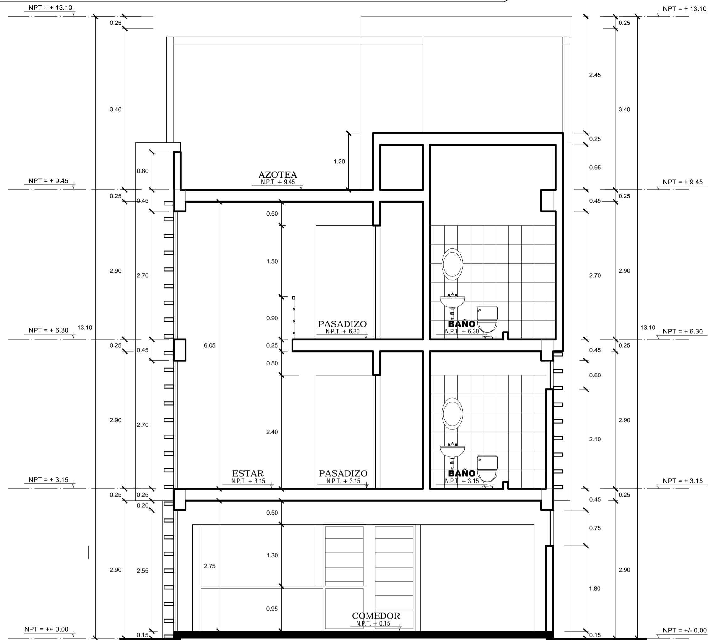
CORTE C - C esc:1/50
