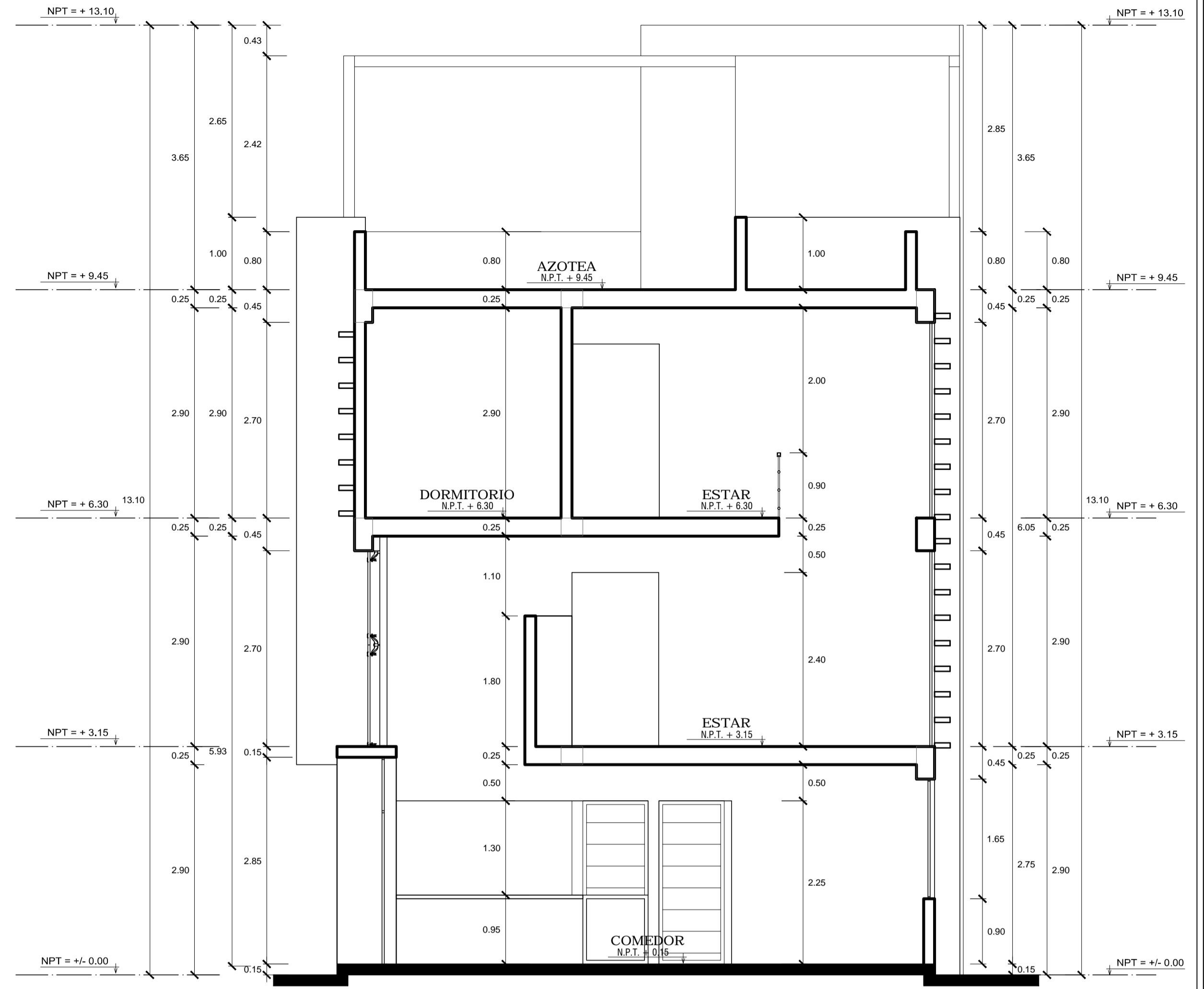
CORTE D - D esc:1/50
