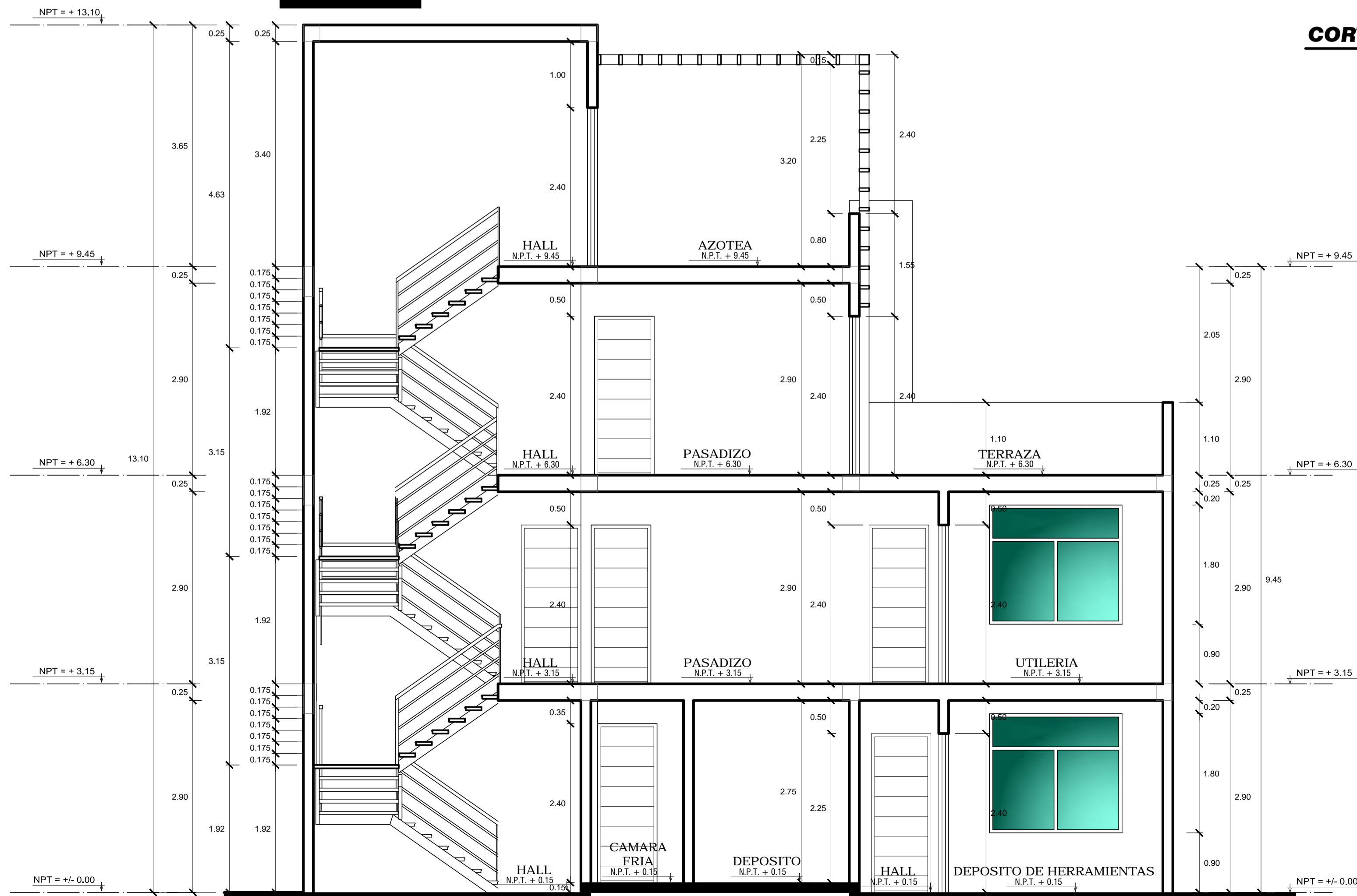
CORTE E - E esc:1/50
