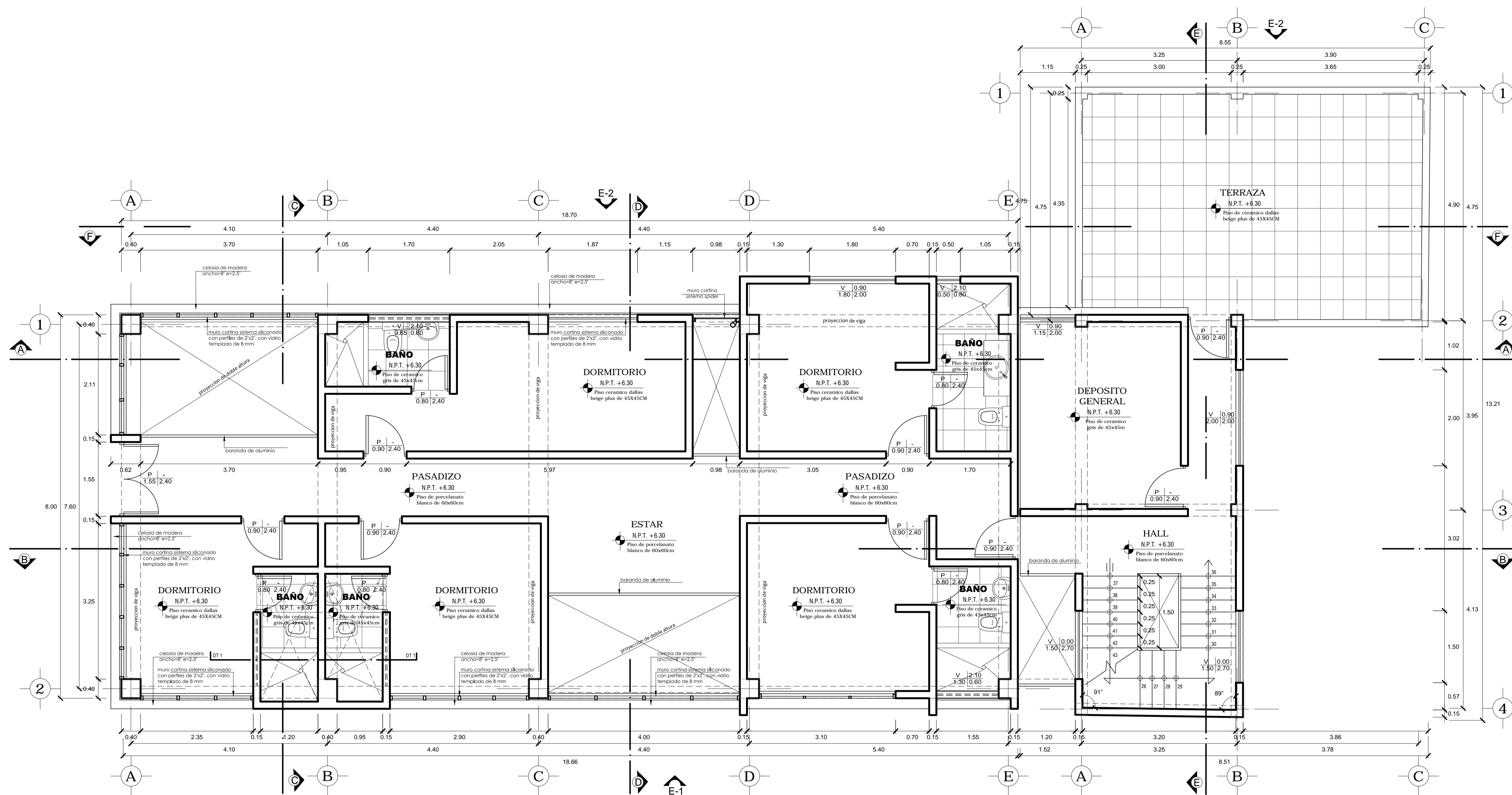
TERCERA PLANTA esc:1/50
