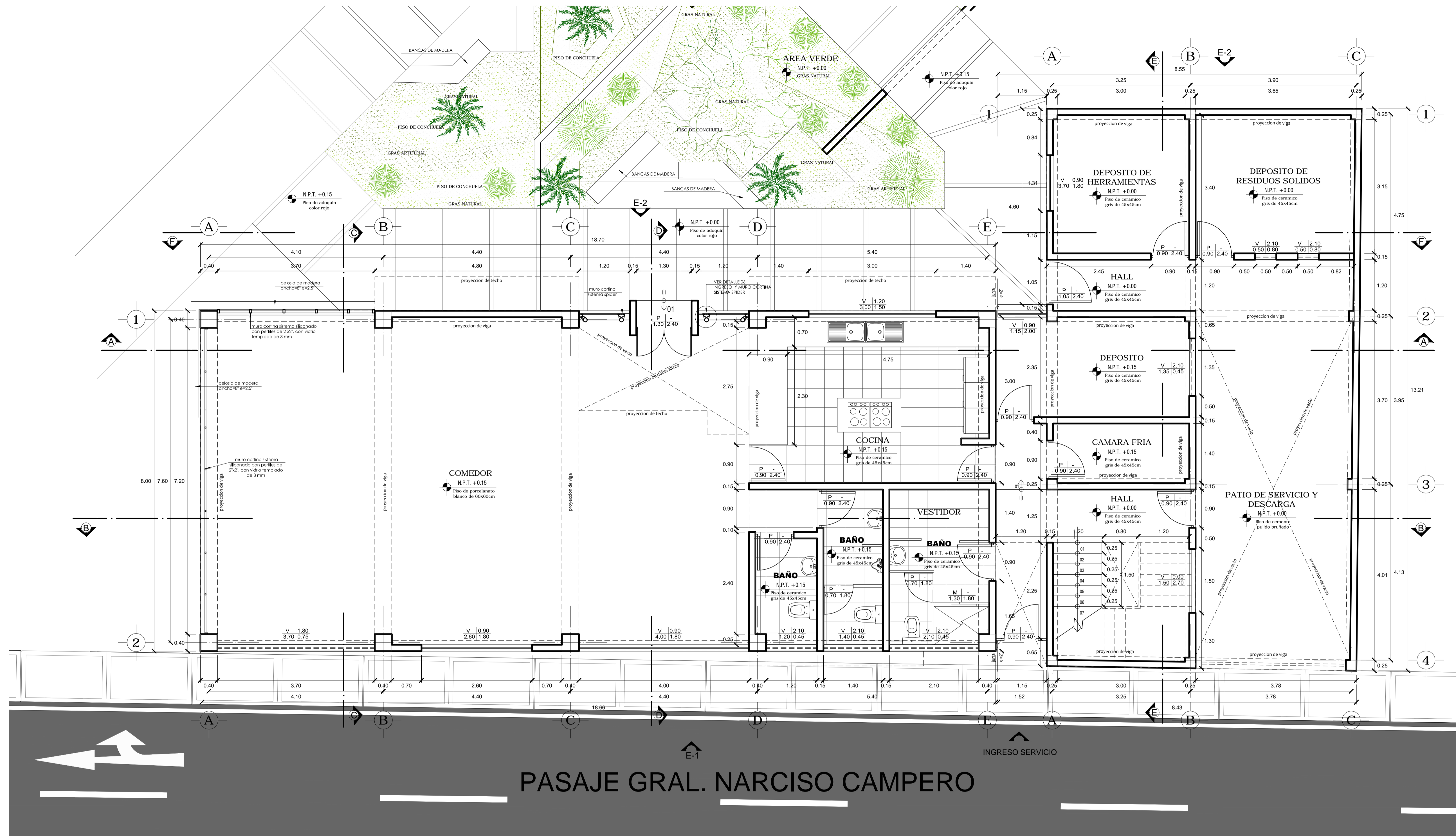
PRIMERA PLANTA esc:1/50
