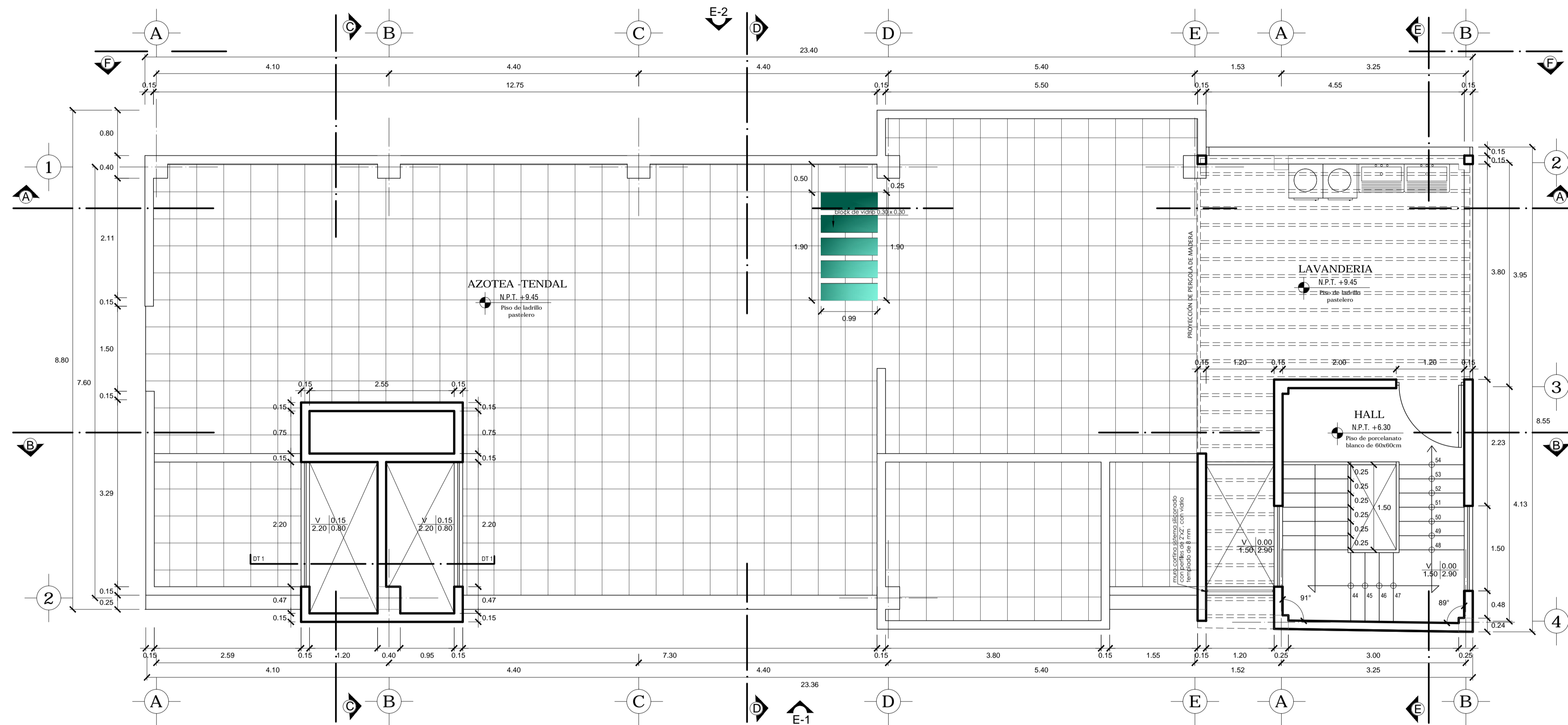
PLANTA DE AZOTEA esc:1/50
