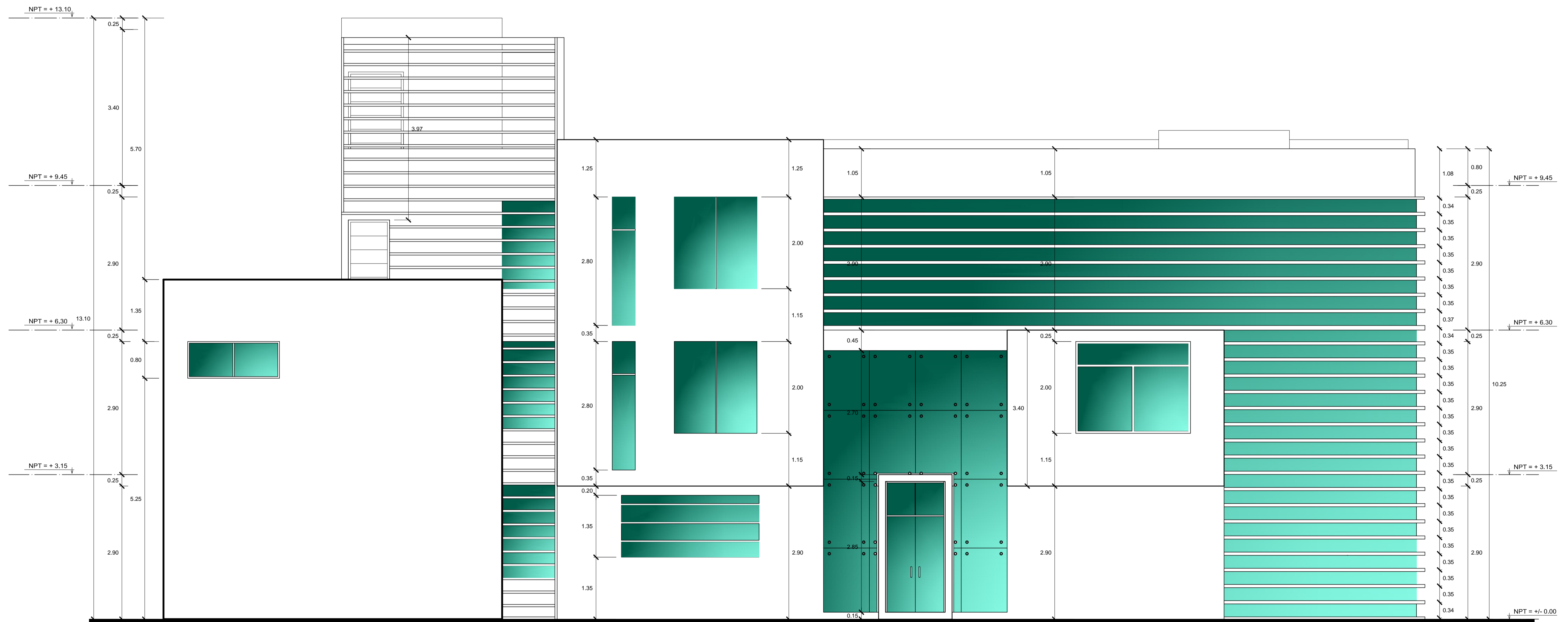
ELEVACION POSTERIOR E-2 esc:1/50
