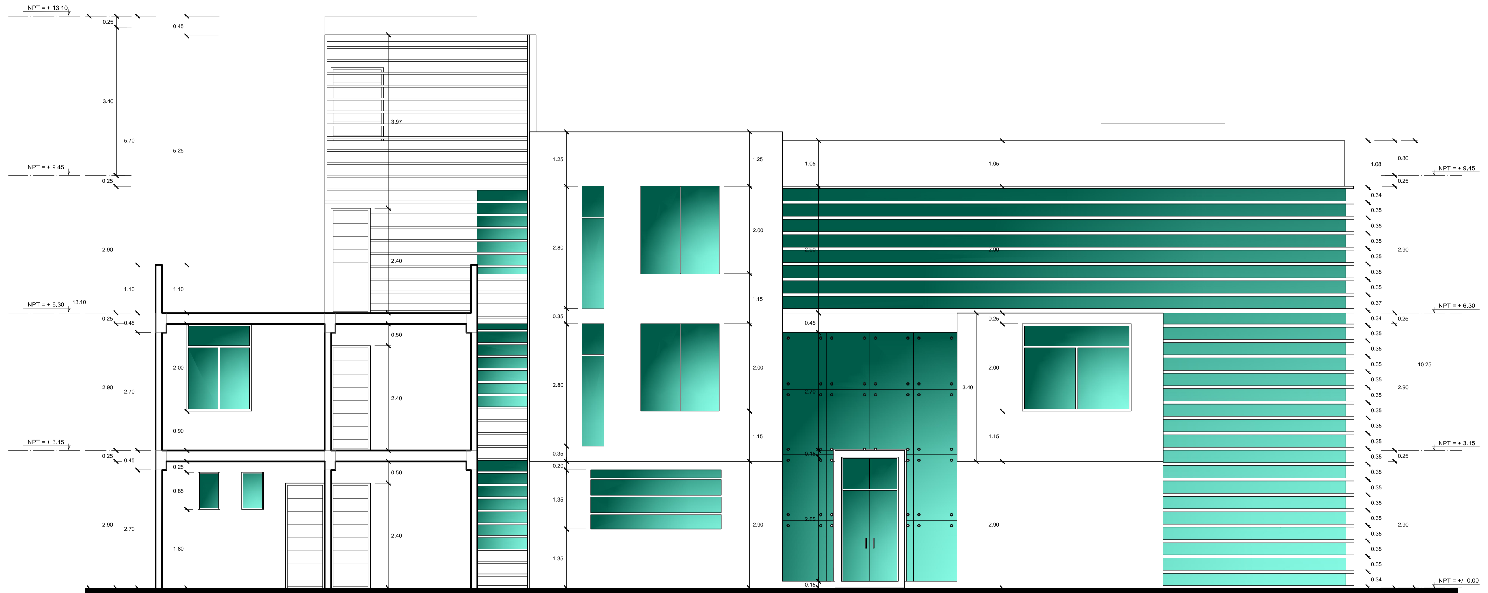
CORTE F - F esc:1/50
