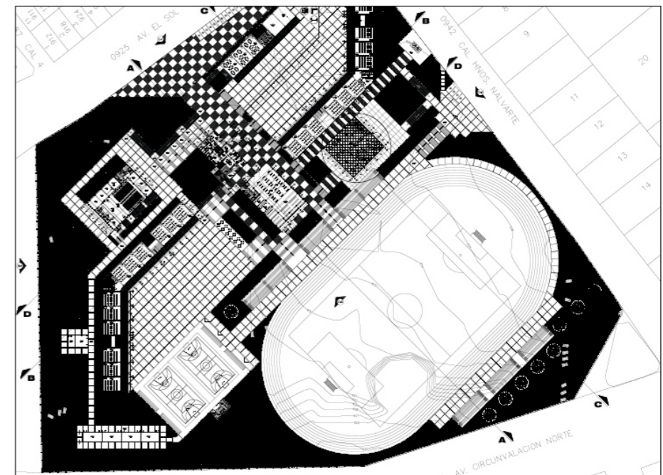
PLANO CLAVE 1° NIVEL - PLANIMETRIA
