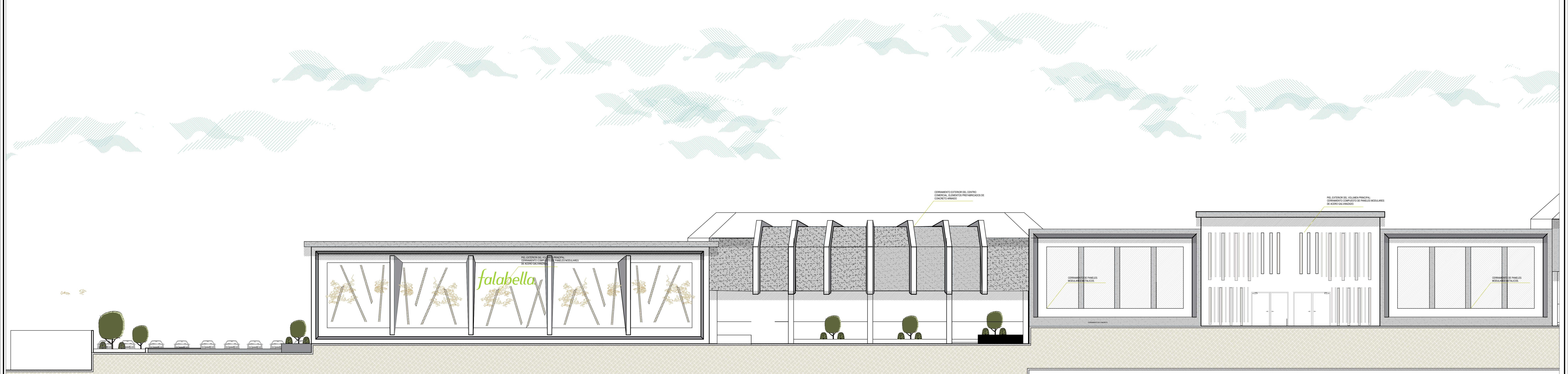
ELEVACION FRONTAL 1-1
