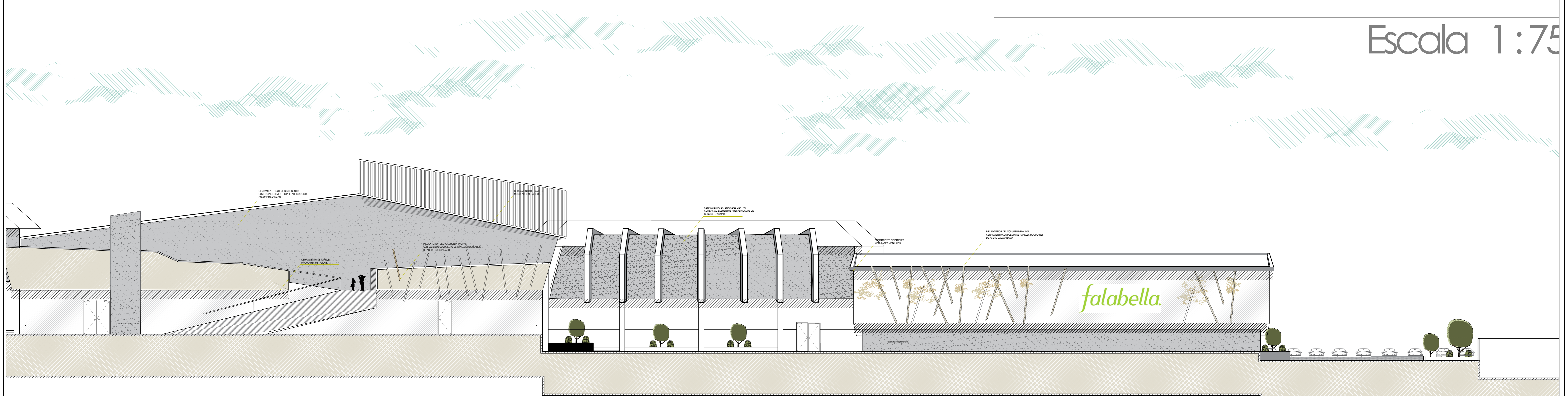
ELEVACION FRONTAL 1-1
