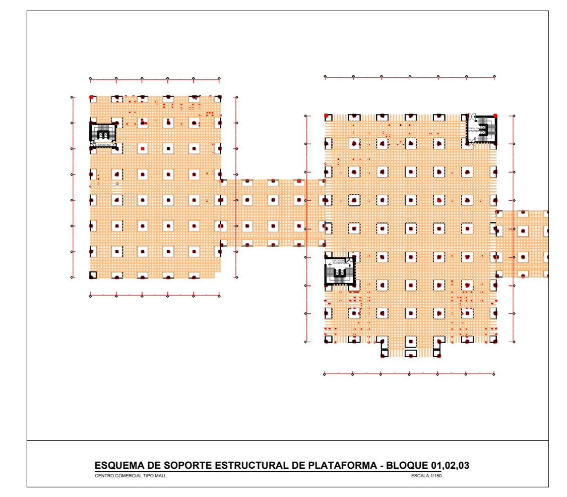
PLANO CLAVE
