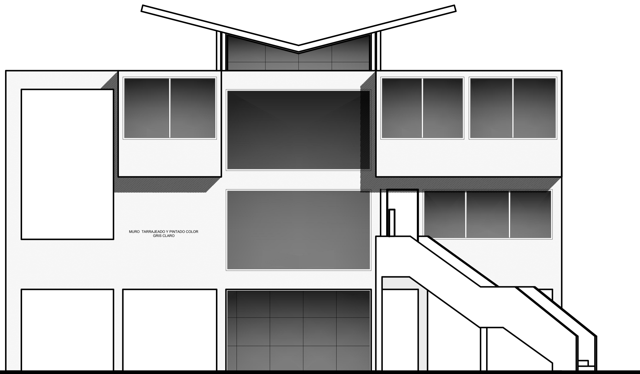
ELEVACIÓN FRONTAL ESCALA: 1/100
