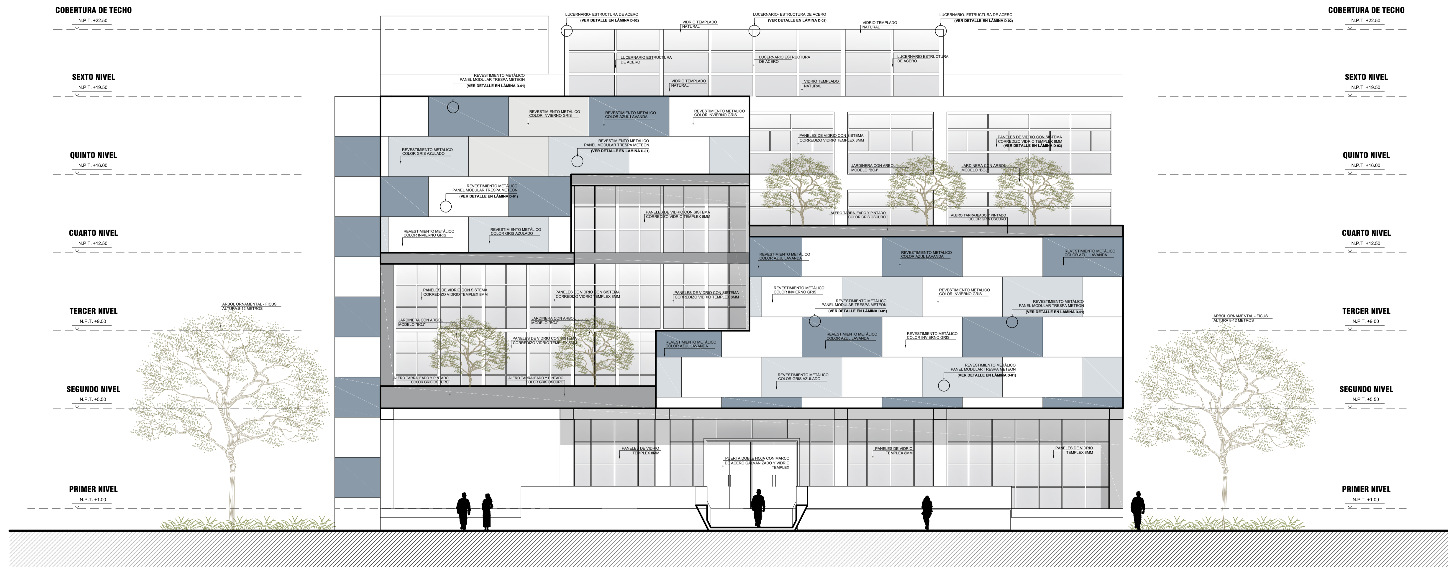
ARQUITECTURA ELEVACIÓN 1 escala : 1/100 Edificio Administrativo de la Universidad Privada de Tacna
