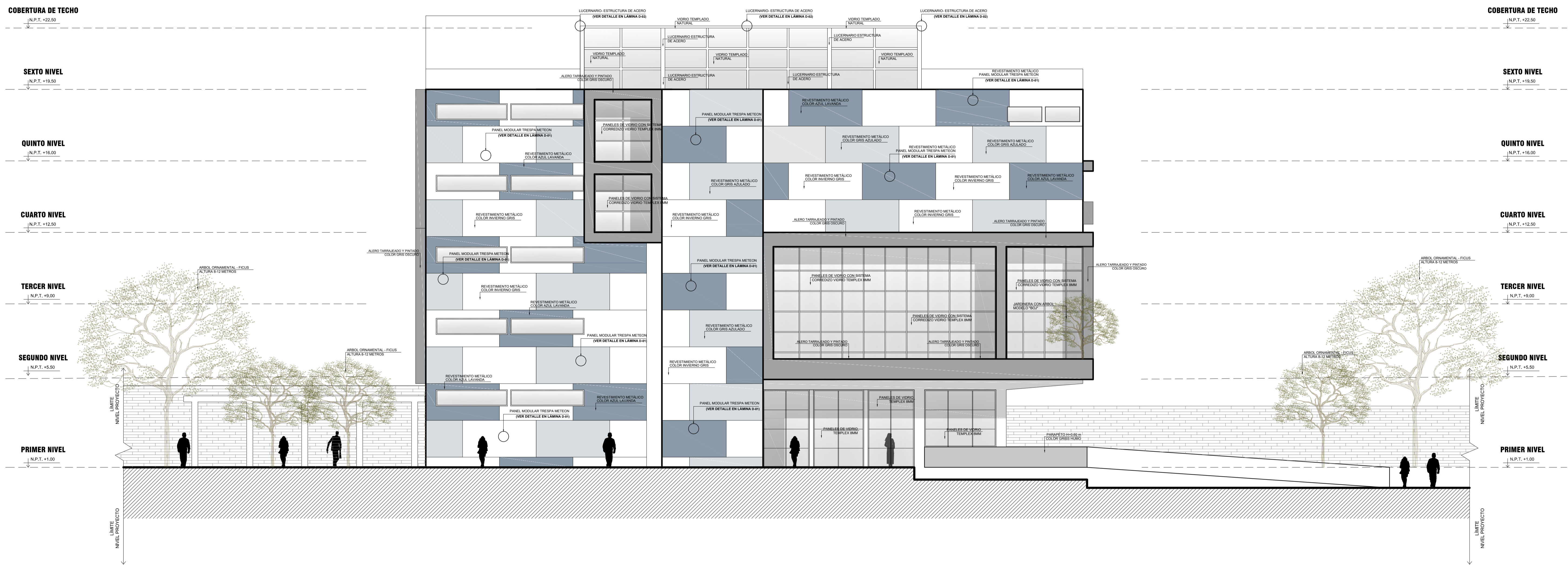
ARQUITECTURA ELEVACIÓN 3 Edificio Administrativo de la Universidad Privada de Tacna escala : 1/100
